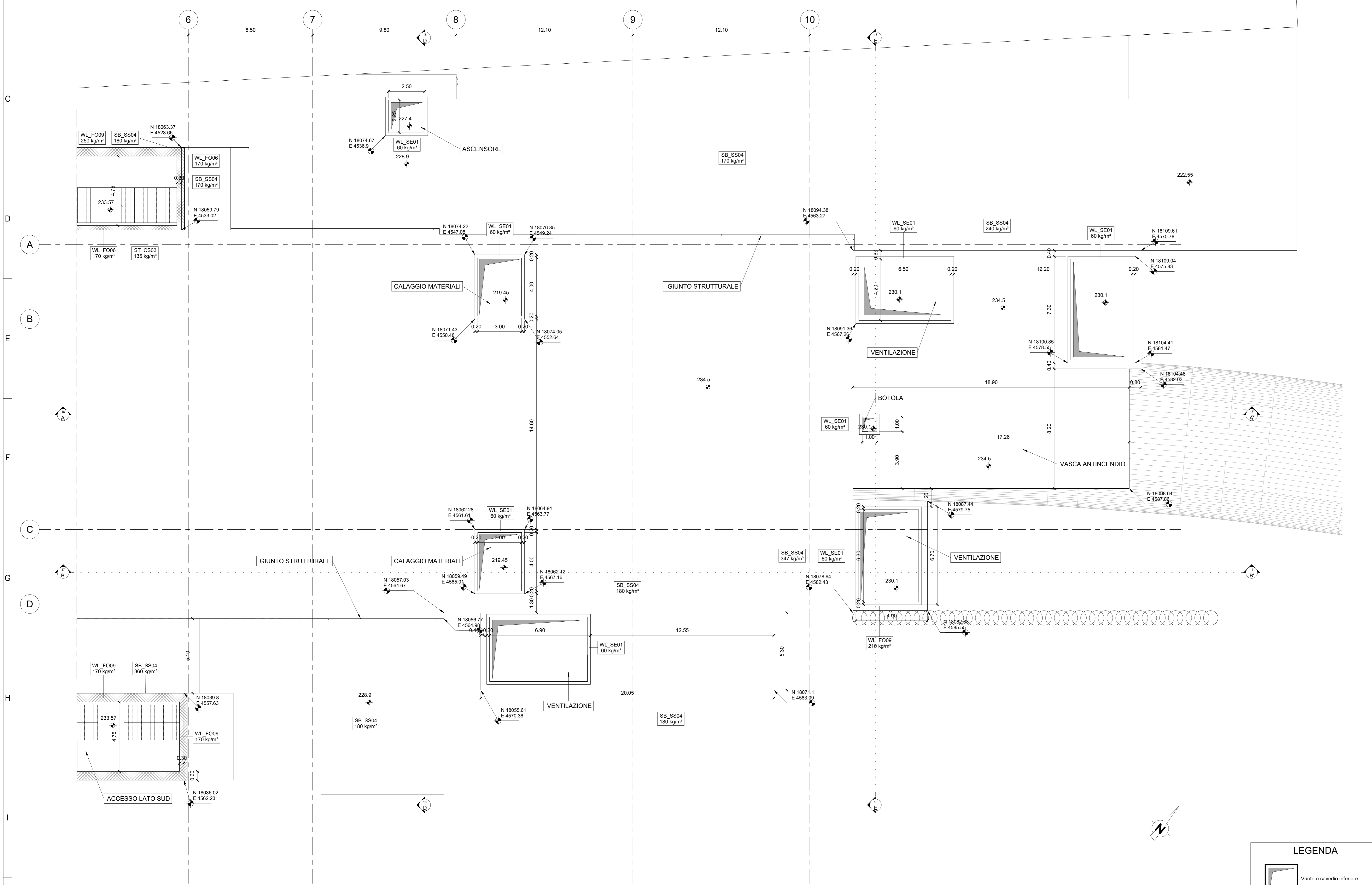
1 PIANTA COPERTURA 2/2 1:100
