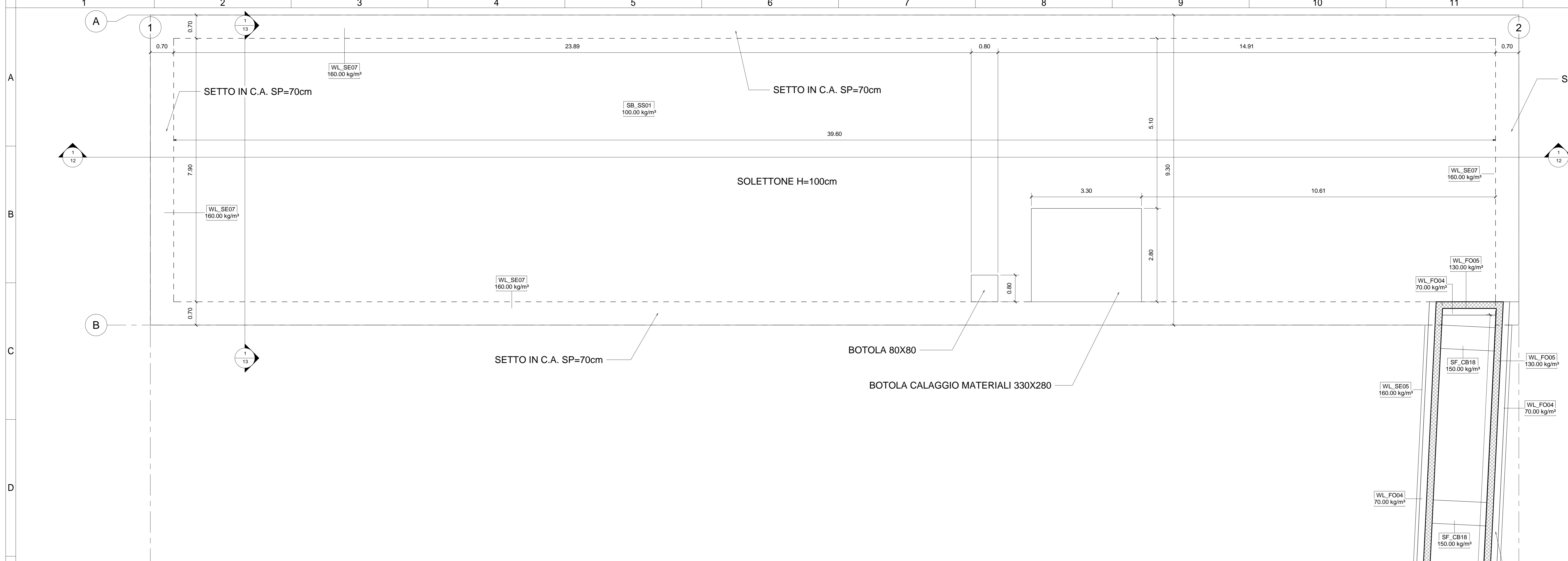
1 Piano copertura (livello 0) 1 : 50
