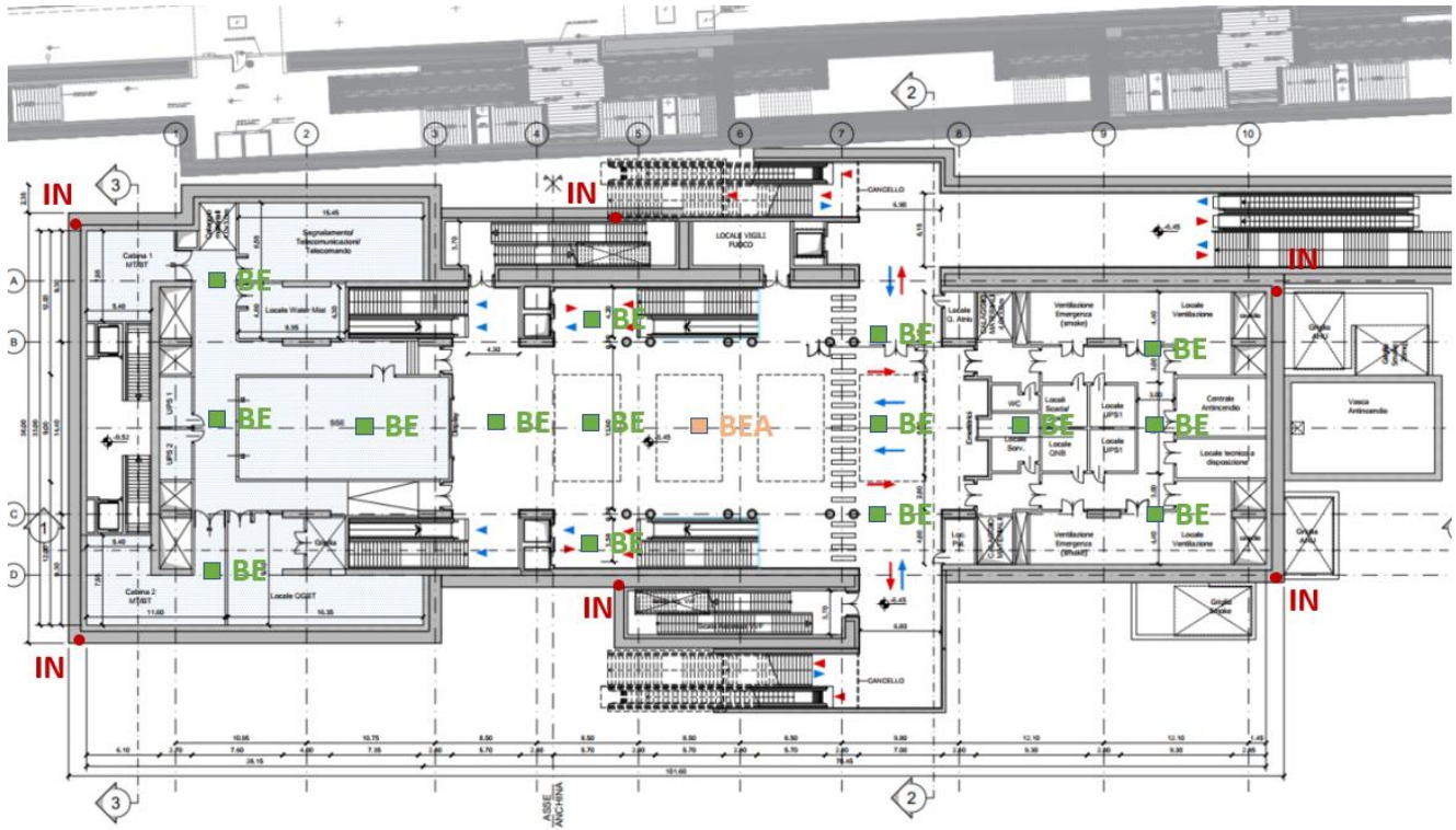
Figura 17. Schema preliminare di monitoraggio – Planimetria tipo
