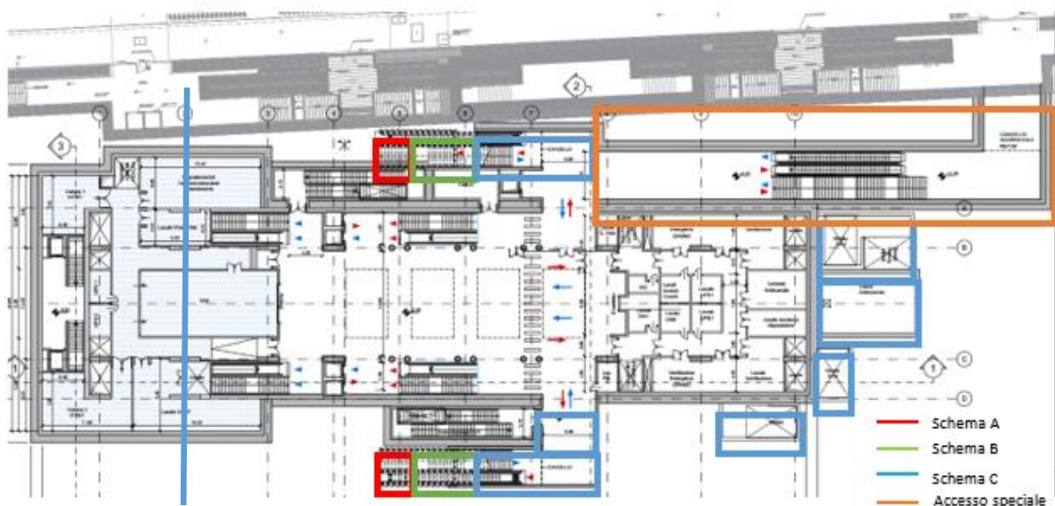
Figura 6. Schema di applicazione sezioni oggetto di analisi
