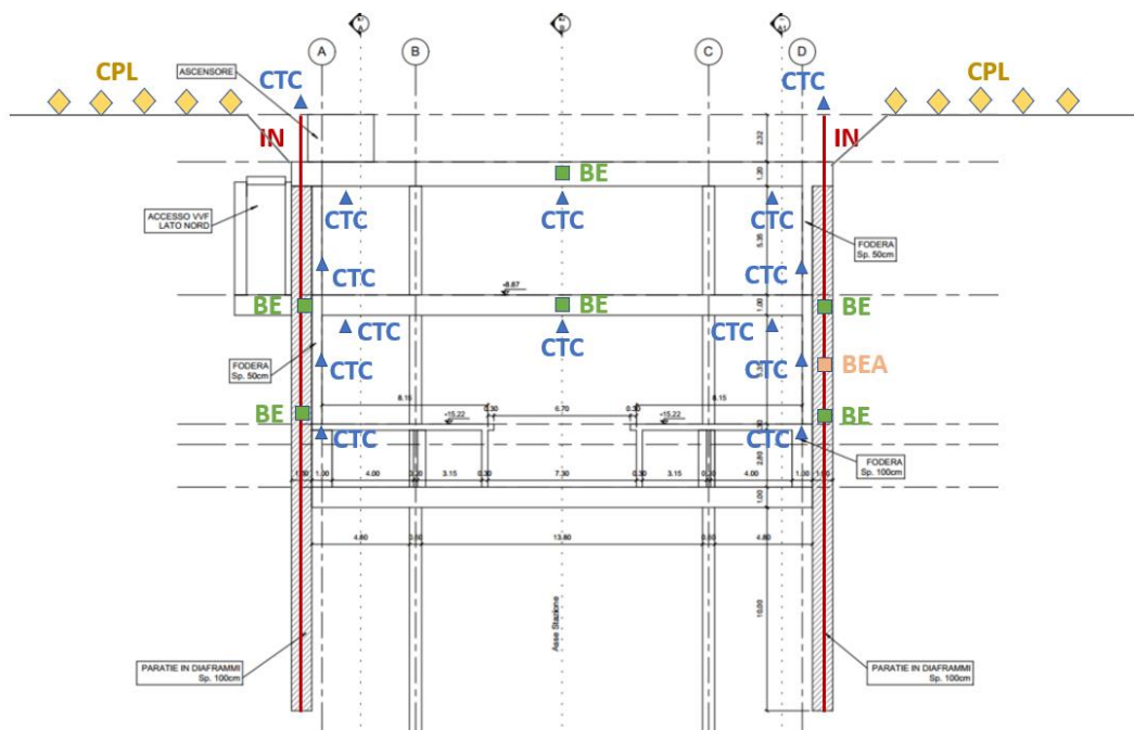
Figura 18. Schema preliminare di monitoraggio – Sezione tipo
