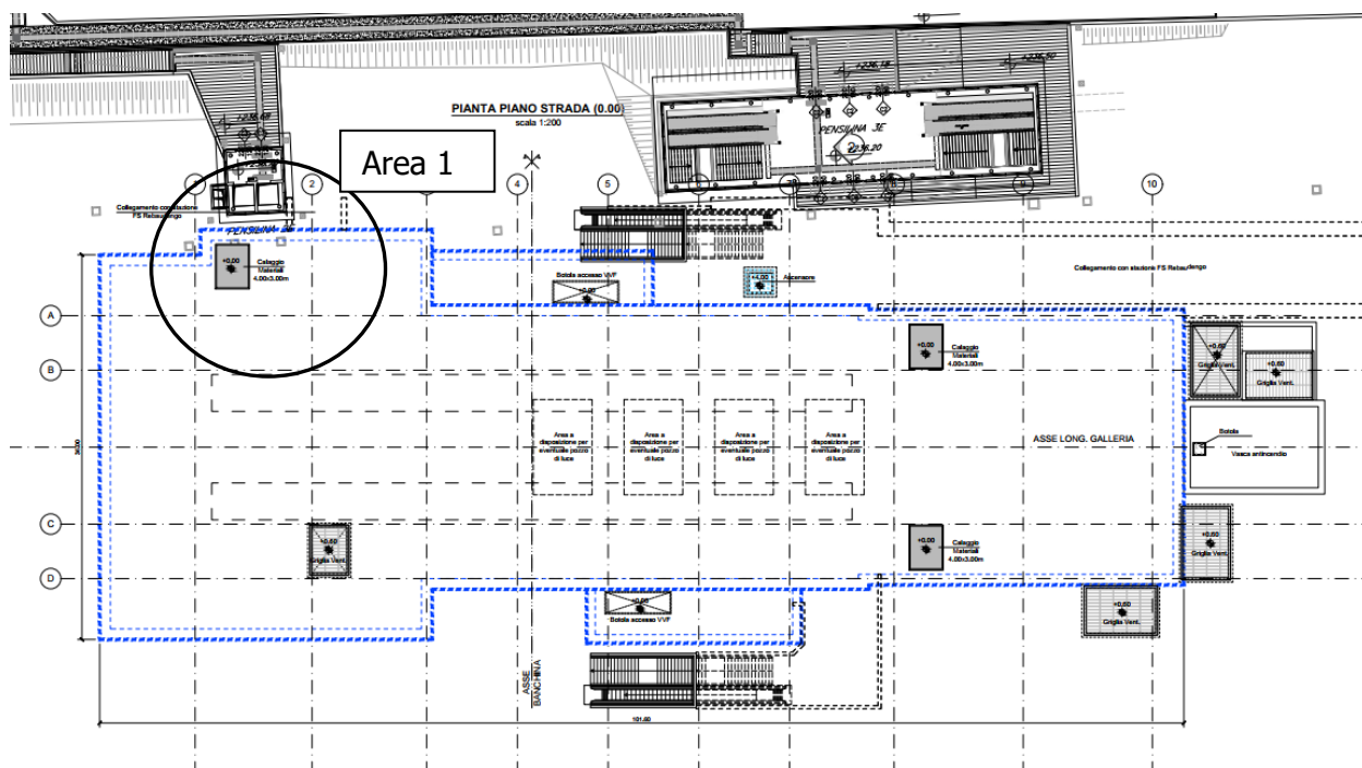
Figura 7. Indicazione sezioni di approfondimento analisi cedimenti
