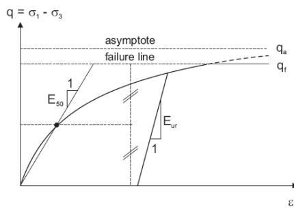
Figura 4. Modello costitutivo Hardening Soil
