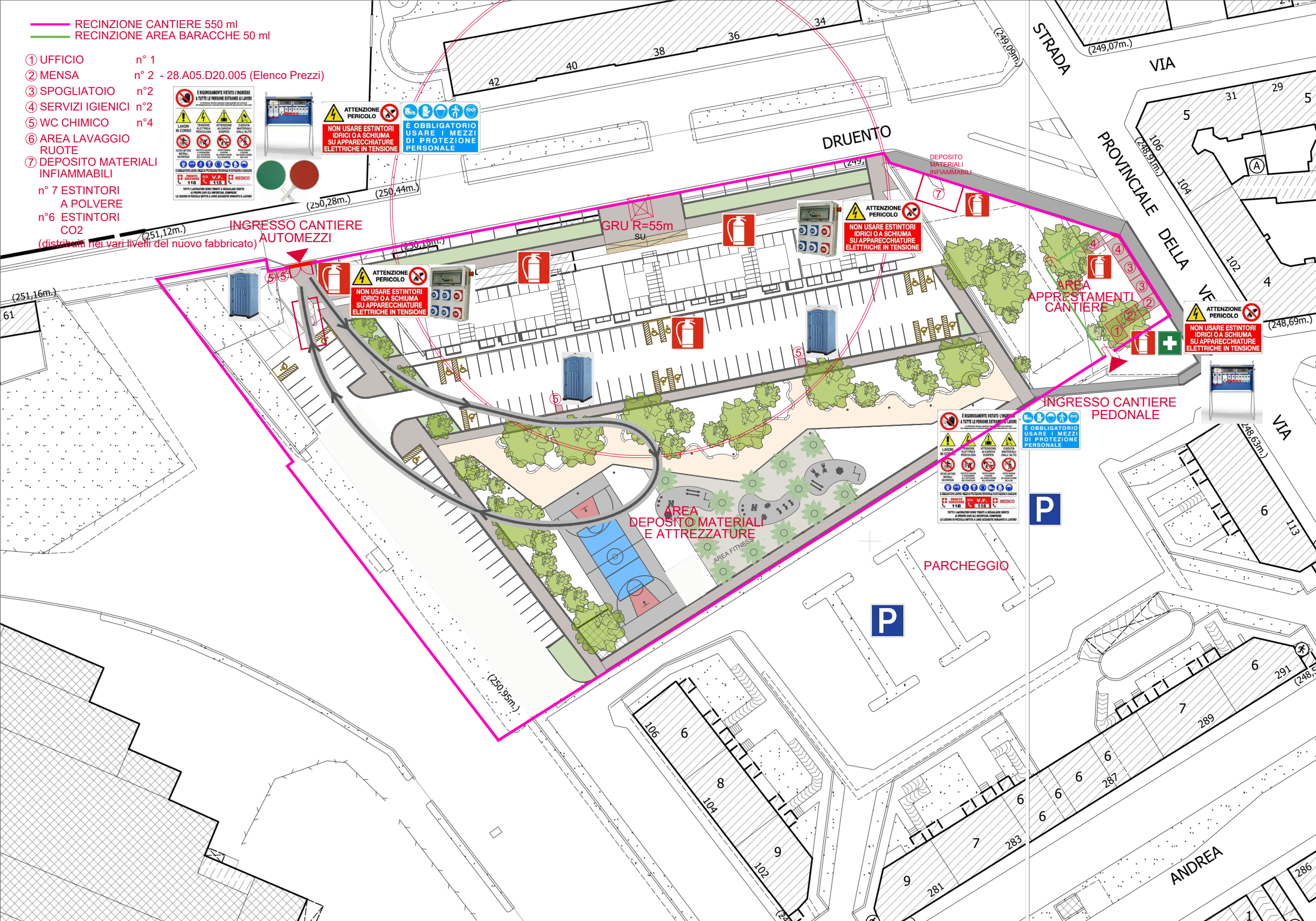
PLANIMETRIA DI CANTIERE FASE 3
