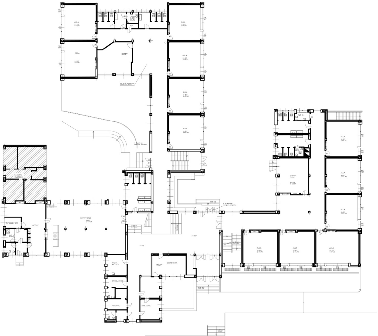
Figura 16 - Pianta piano terra
