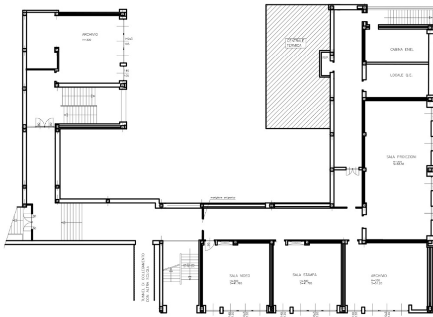
Figura 15 - Pianta piano seminterrato
