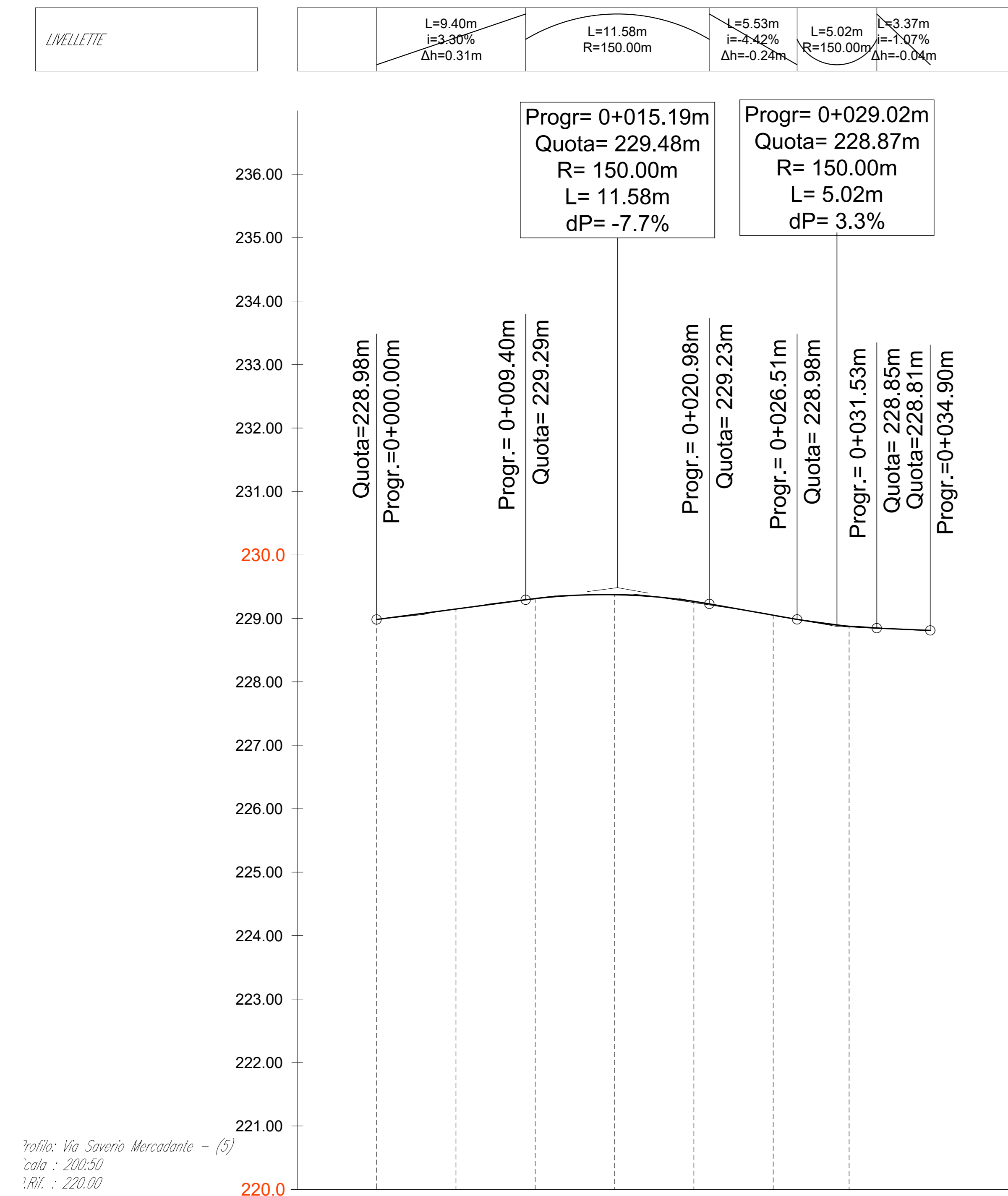
Profilo longitudinale | scala 1:200
