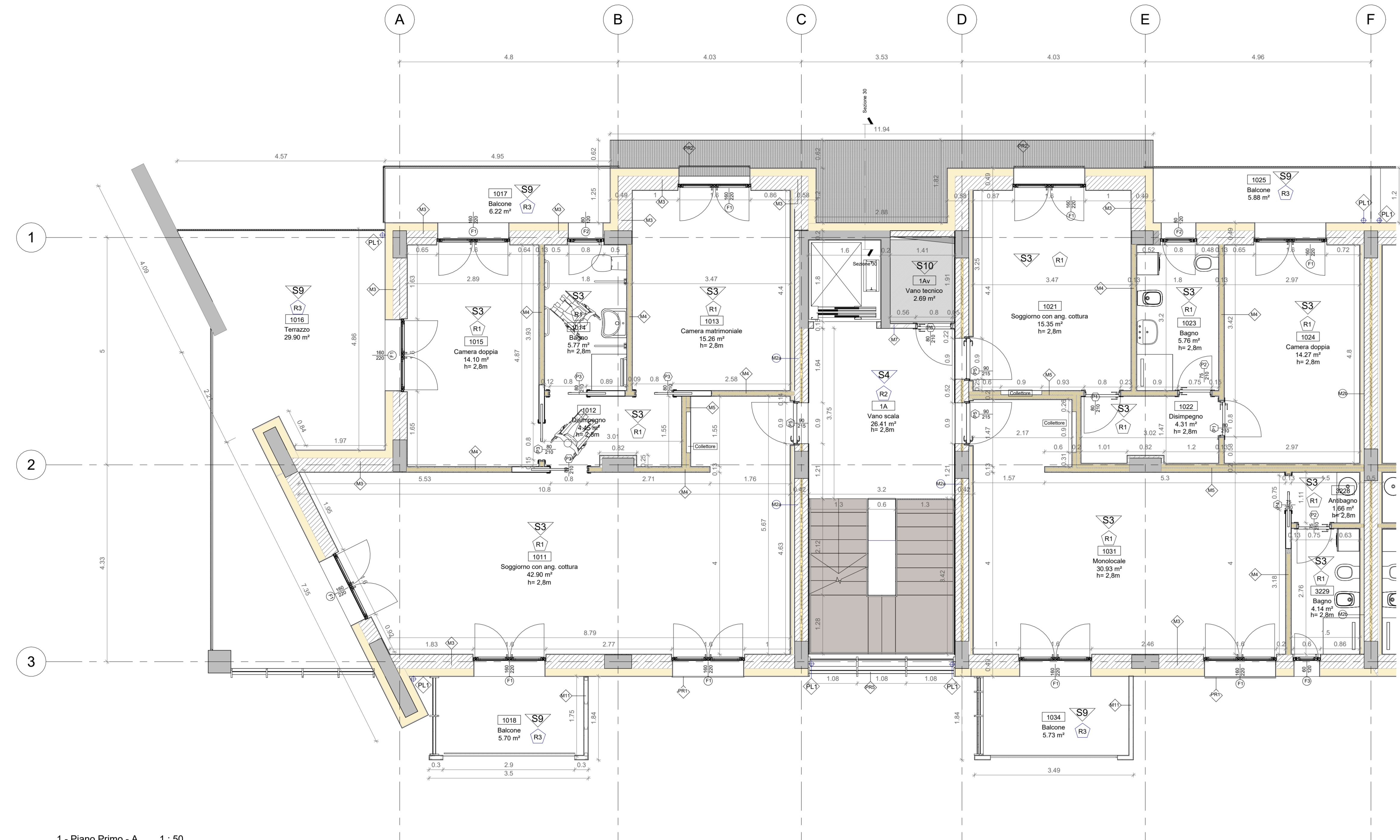
1 - Piano Primo - A 1:50
