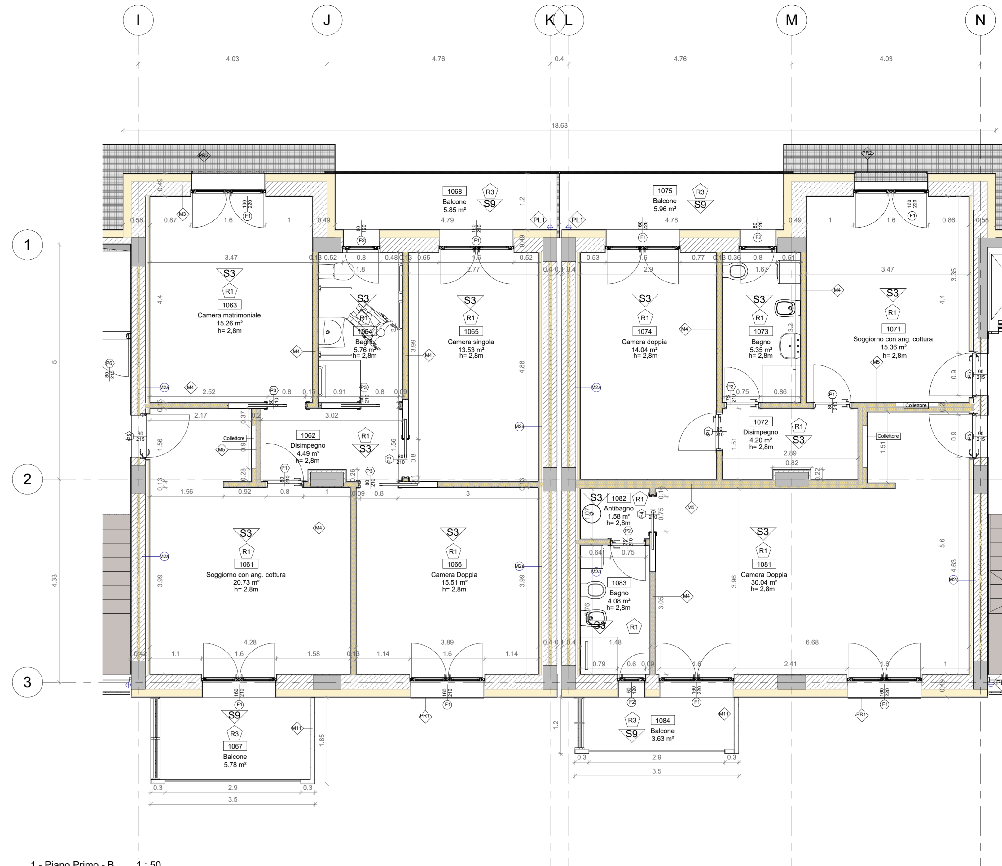
1 - Piano Primo - B 1:50
