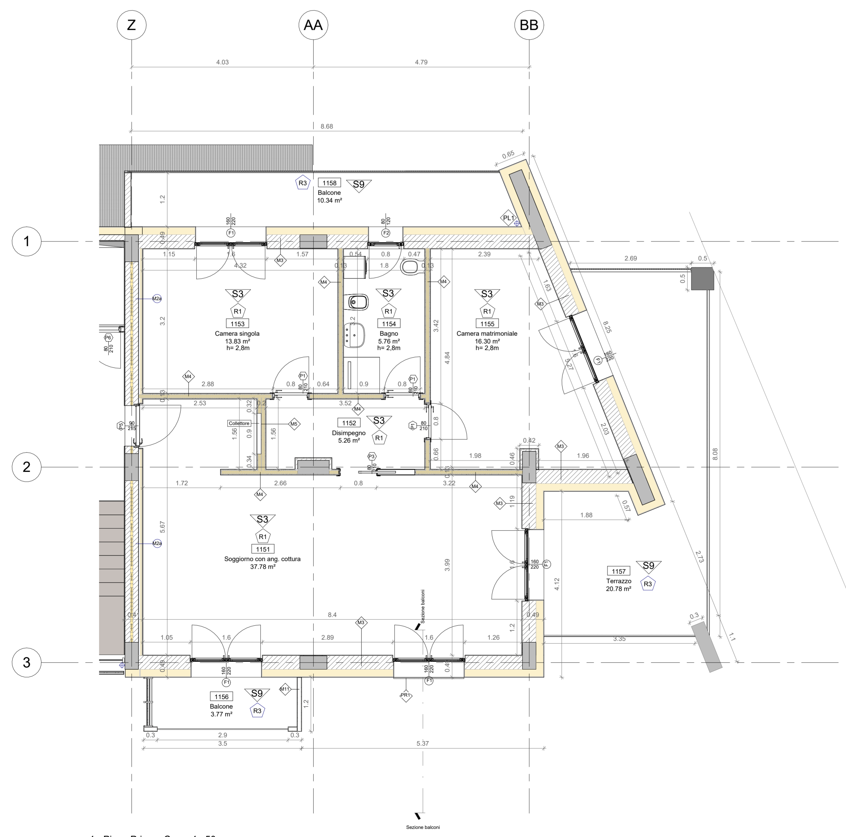
1 - Piano Primo - C 1:50
