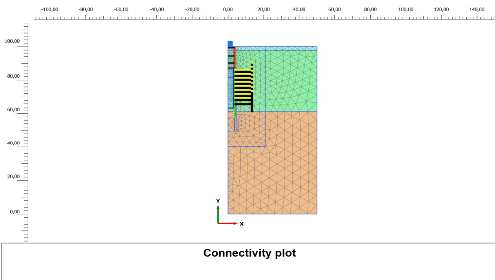
Figura 4. Modello di calcolo e relativa mesh del pozzo Politecnico“PPO”
