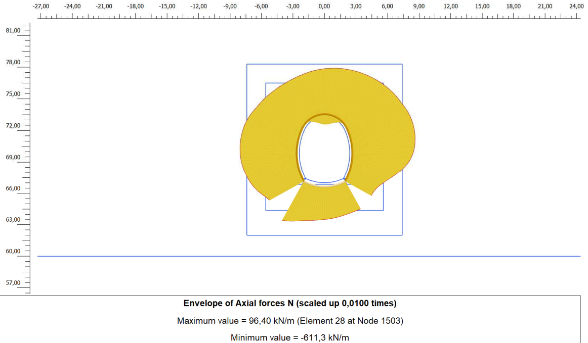
Figura 24. Involuppo diagramma dello sforzo normale – rivestimento definitivo: Azione sismica (-)
