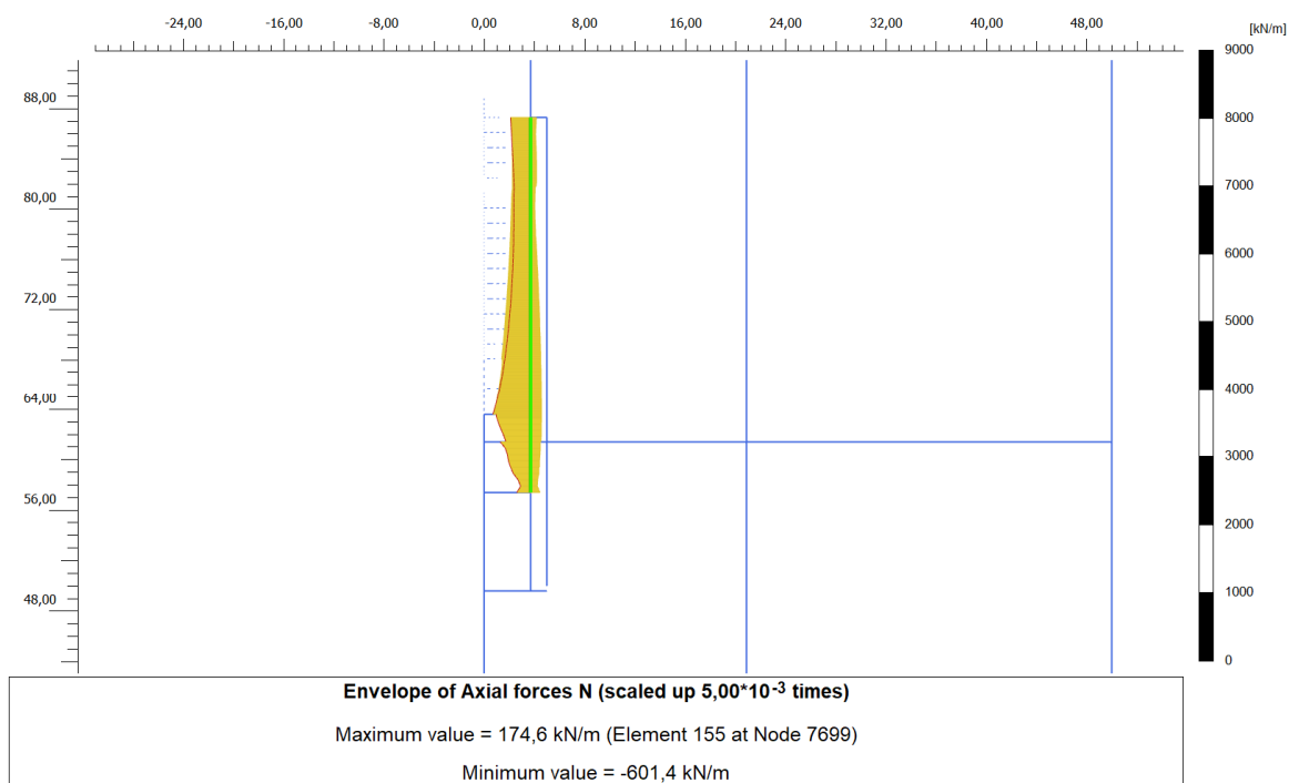
Figura 13. Involuppo dello sforzo normale – SLE
