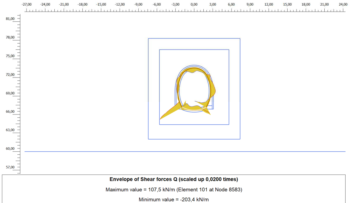
Figura 25. Involuppo diagramma del taglio – rivestimento definitivo: Azione sismica (-)
