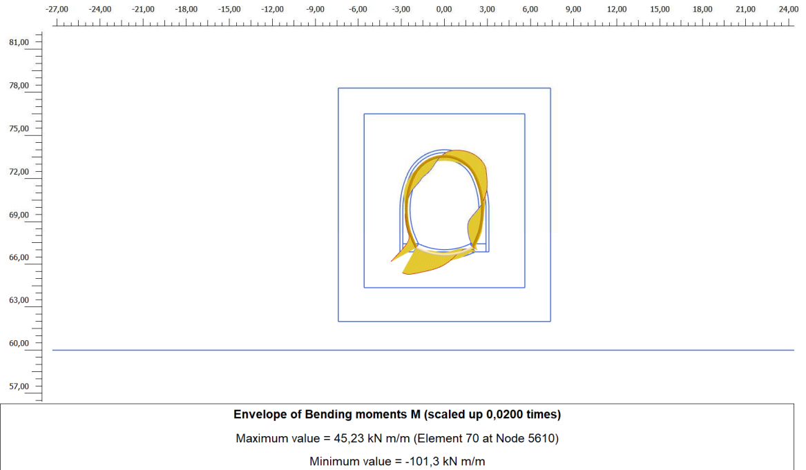
Figura 26. Involuppo diagramma del momento flettente – rivestimento definitivo: Azione sismica (-)
