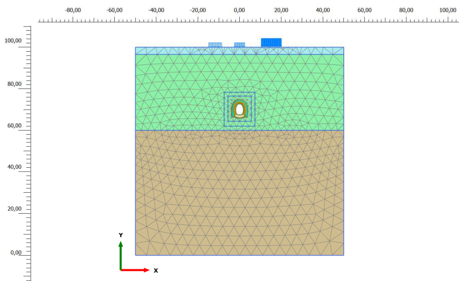
Figura 5. Modello di calcolo e relativa mesh del tronchino di collegamento del pozzo Politecnico“PPO”
