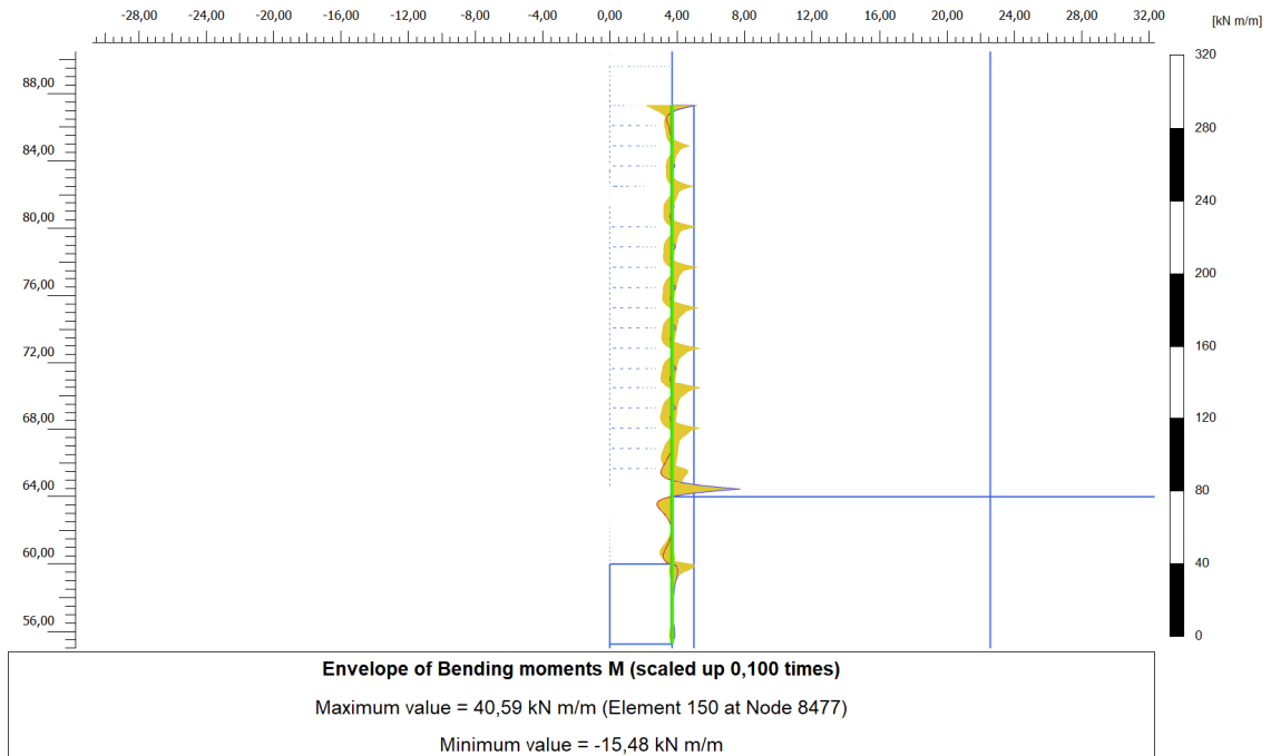
Figura 9. Involuppo di momento flettente – SLE
