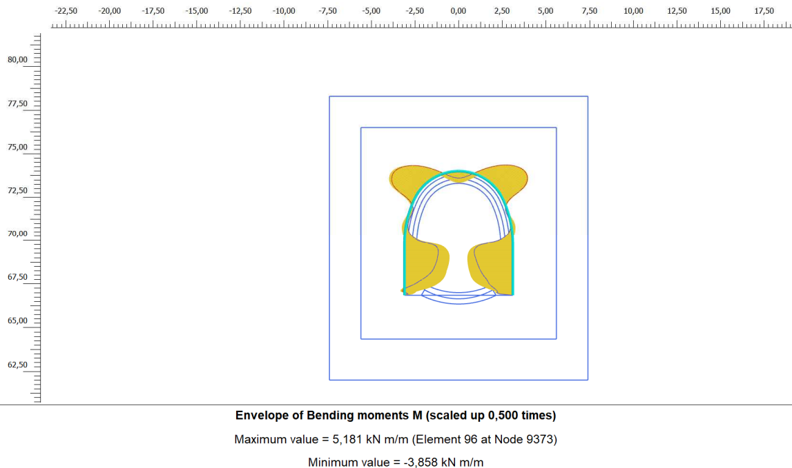
Figura 14. Inviluppo diagramma del momento flettente - centine
