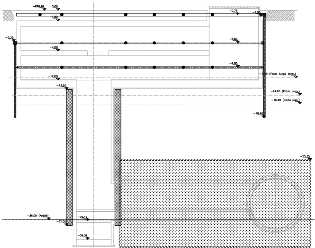
Figura 2. Sezione longitudinale del pozzo di ventilazione Porta Nuova (PPN)
