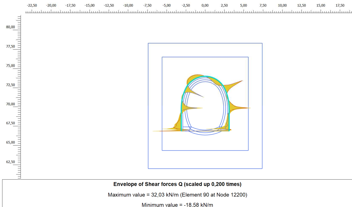
Figura 15. Inviluppo diagramma del taglio – centine
