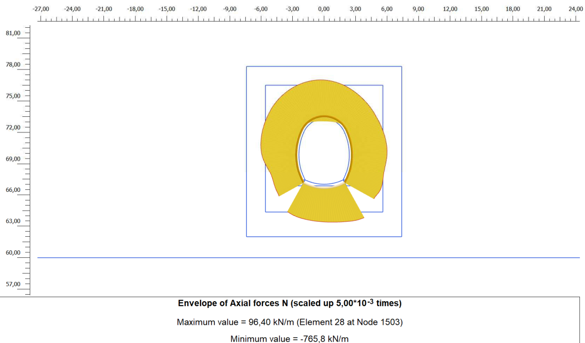
Figura 19. Involuppo diagramma dello sforzo normale – rivestimento definitivo: Azione sismica (+)
