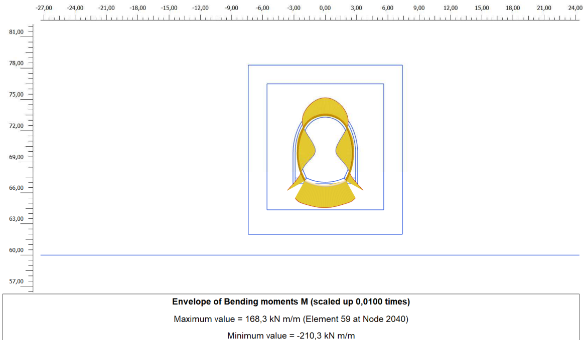
Figura 18. Inviluppo diagramma del momento flettente – Rivestimento definitivo: fase di falda a lungo termine
