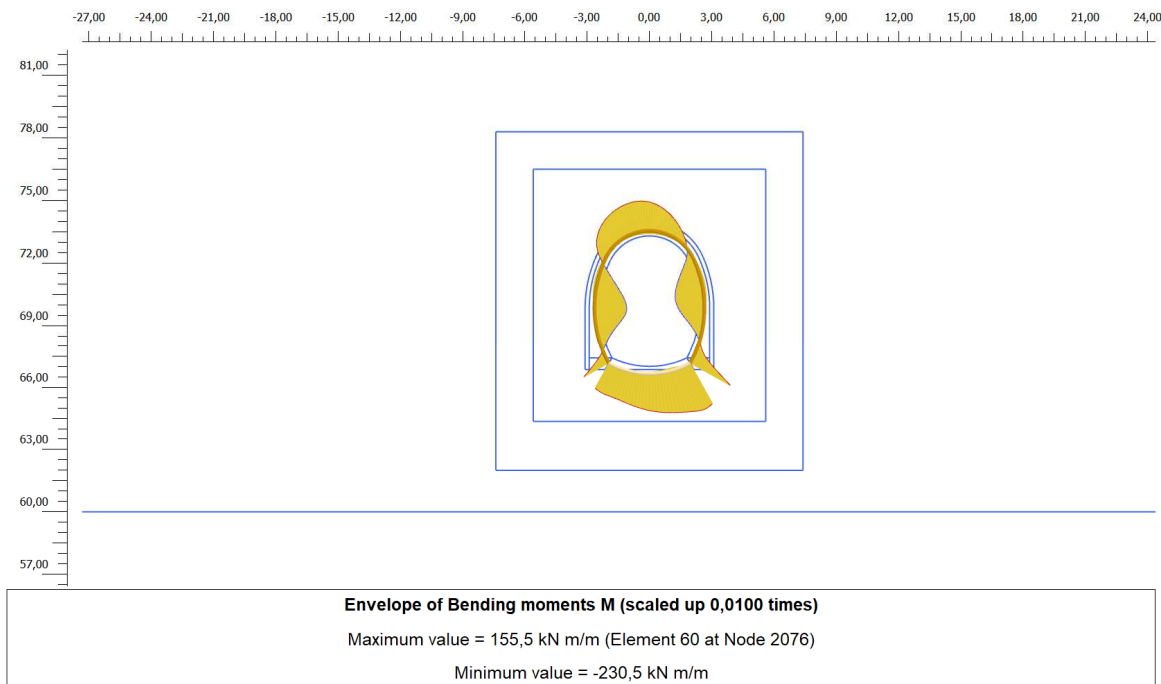
Figura 21. Inviluppo diagramma del momento flettente – rivestimento definitivo: Azione sismica (+)
