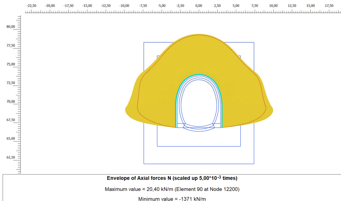
Figura 13. Involuppo diagramma dello sforzo normale - centine
