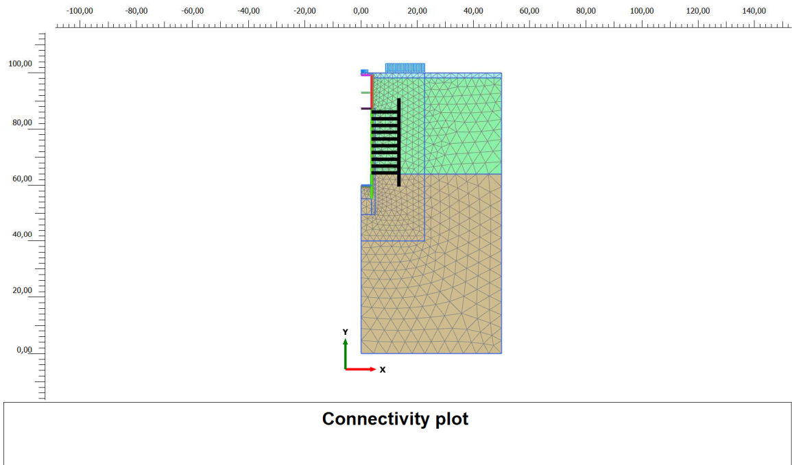
Figura 5. Modello di calcolo e relativa mesh del pozzo Portanuova "PPN"
