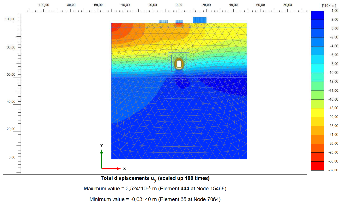
Figura 27. Campo dei cedimenti fase azione sismica (-)
