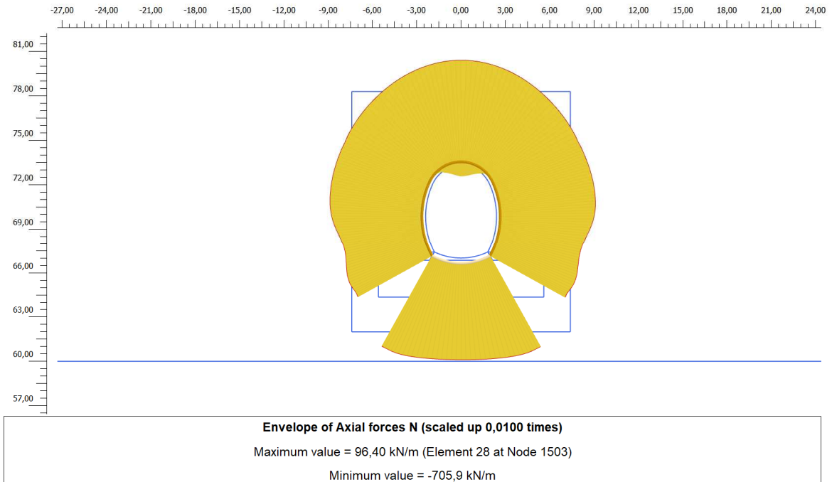
Figura 16. Involuppo diagramma dello sforzo normale – rivestimento definitivo: Fase di falda a lungo termine
