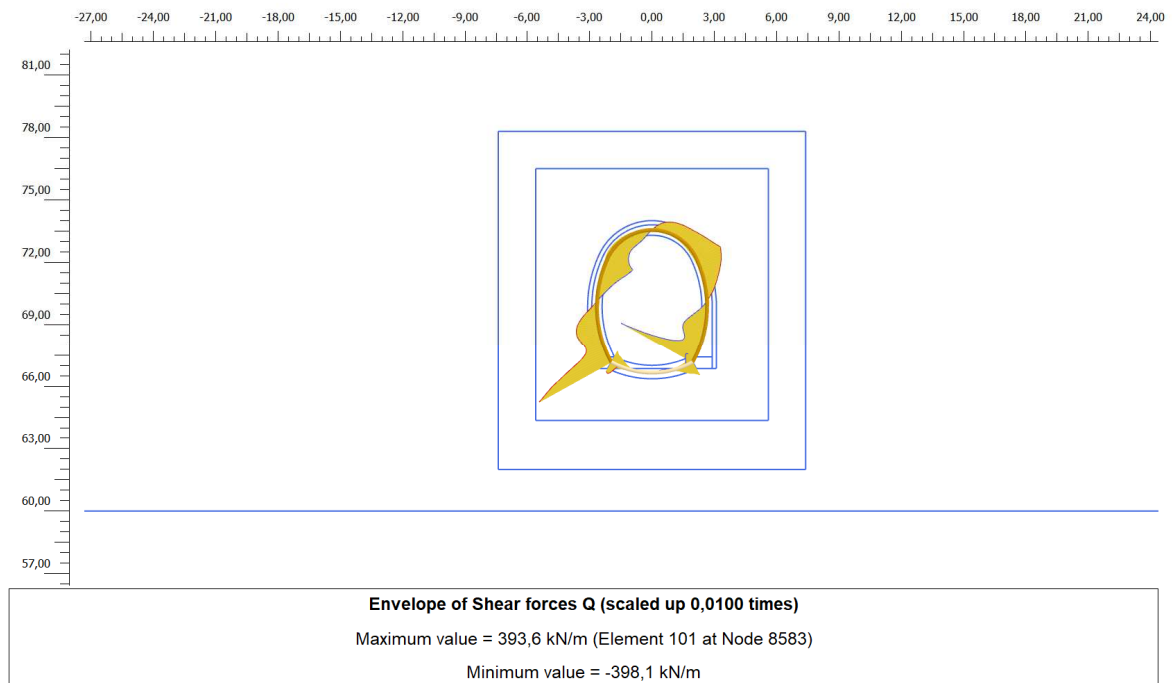
Figura 17. Involuppo diagramma del taglio – rivestimento definitivo: Fase di falda a lungo termine
