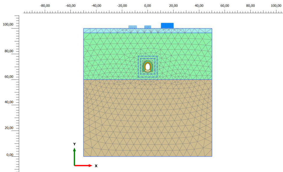
Figura 6. Modello di calcolo e relativa mesh del tronchino di collegamento del pozzo Portanuova "PPN"
