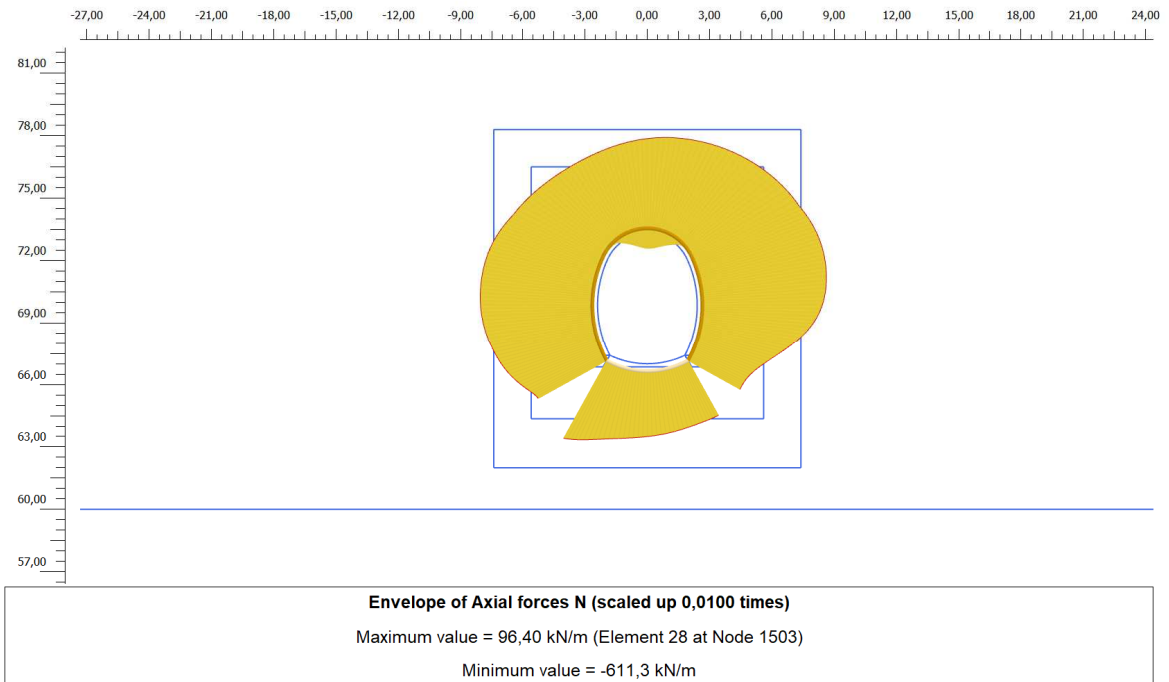
Figura 22. Involuppo diagramma dello sforzo normale – rivestimento definitivo: Azione sismica (-)
