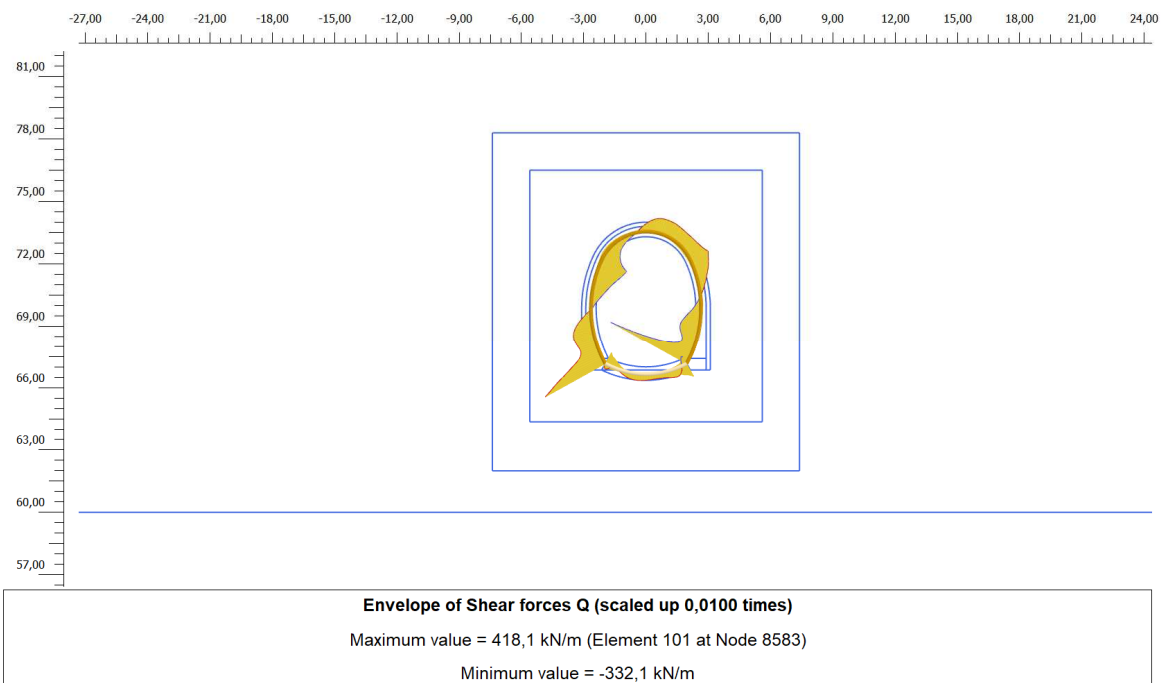
Figura 20. Inviluppo diagramma del taglio – rivestimento definitivo: Azione sismica (+)
