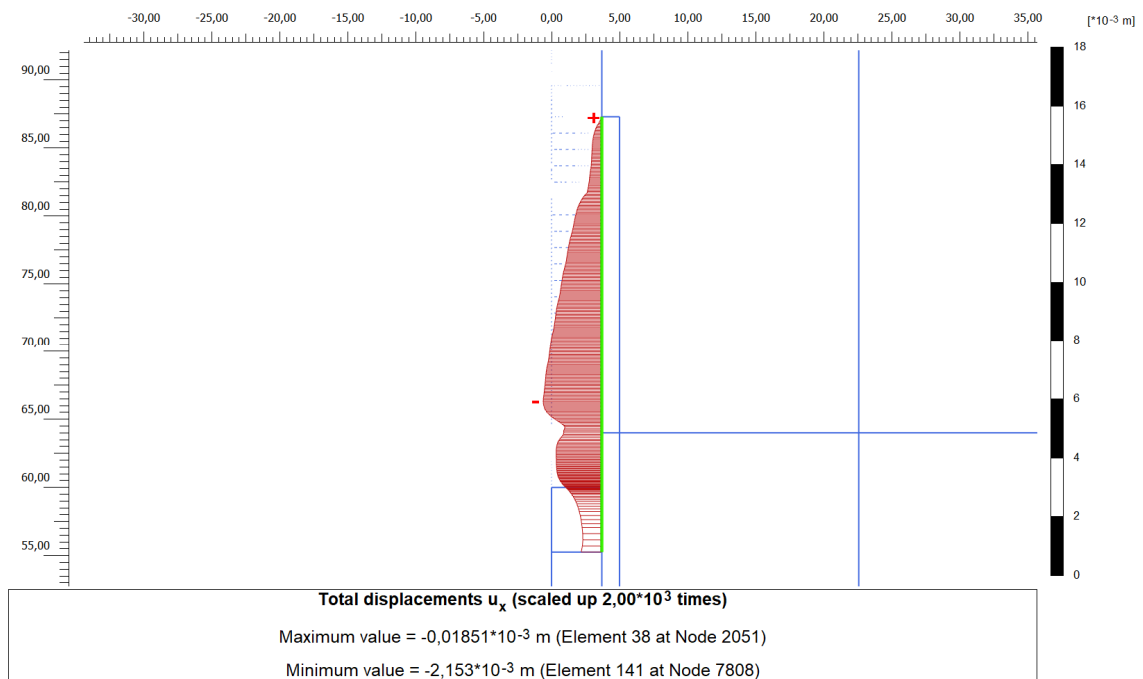
Figura 12. Diagramma degli spostamenti orizzontali della paratia
