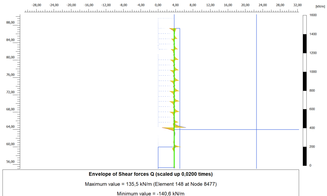
Figura 10. Involuppo di taglio – SLE
