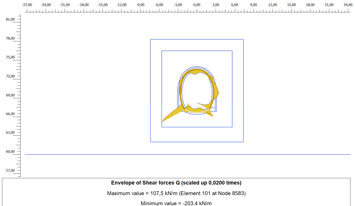
Figura 23. Inviluppo diagramma del taglio – rivestimento definitivo: Azione sismica (-)
