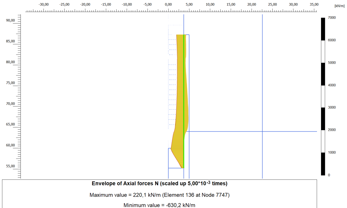
Figura 11. Involuppo dello sforzo normale – SLE
