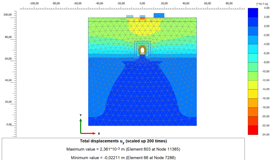
Figura 25. Campo dei cedimenti fase di falda a lungo termine
