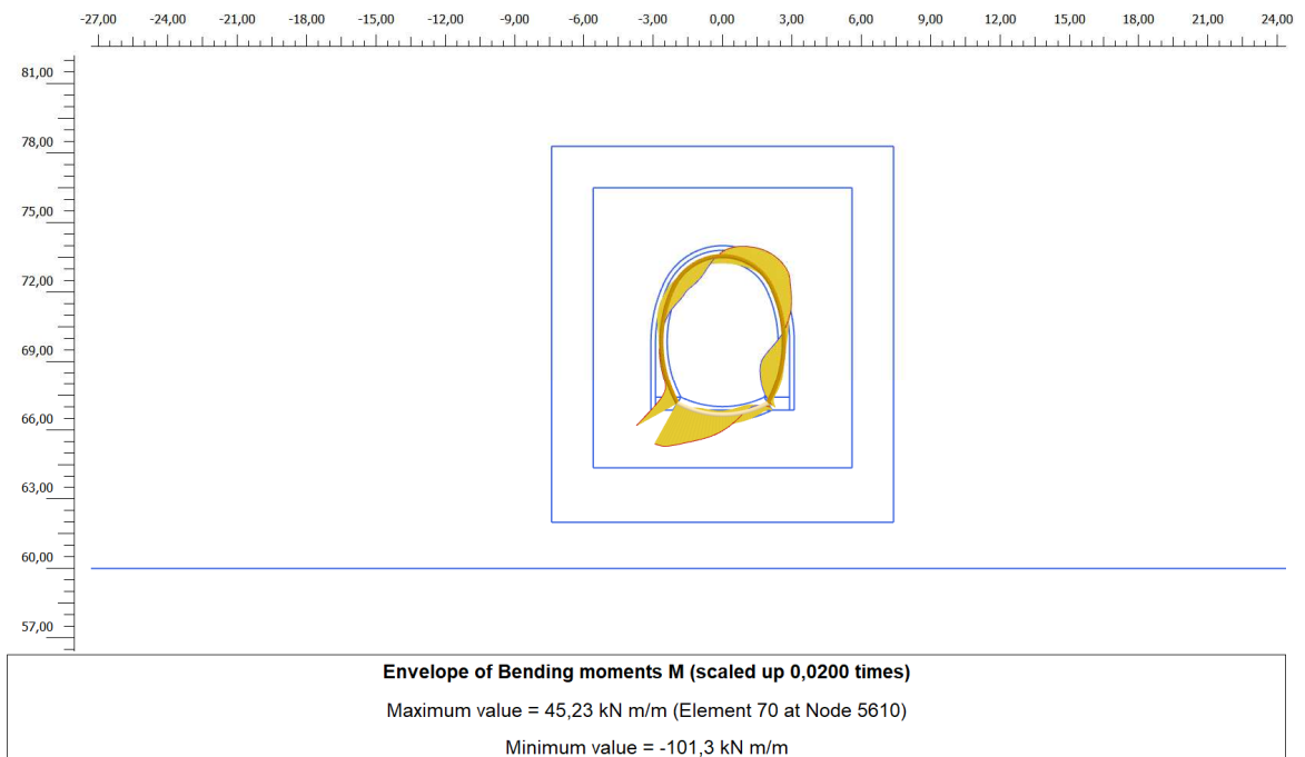
Figura 24. Inviluppo diagramma del momento flettente – rivestimento definitivo: Azione sismica (-)
