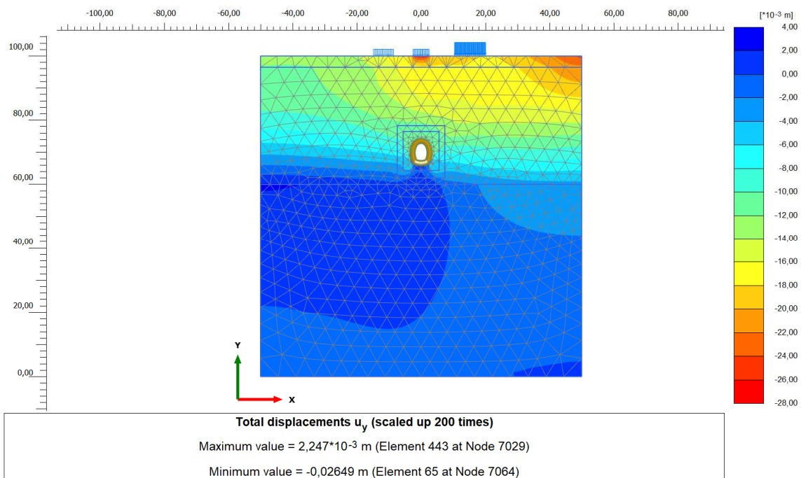
Figura 25. Campo dei cedimenti fase azione sismica (+)
