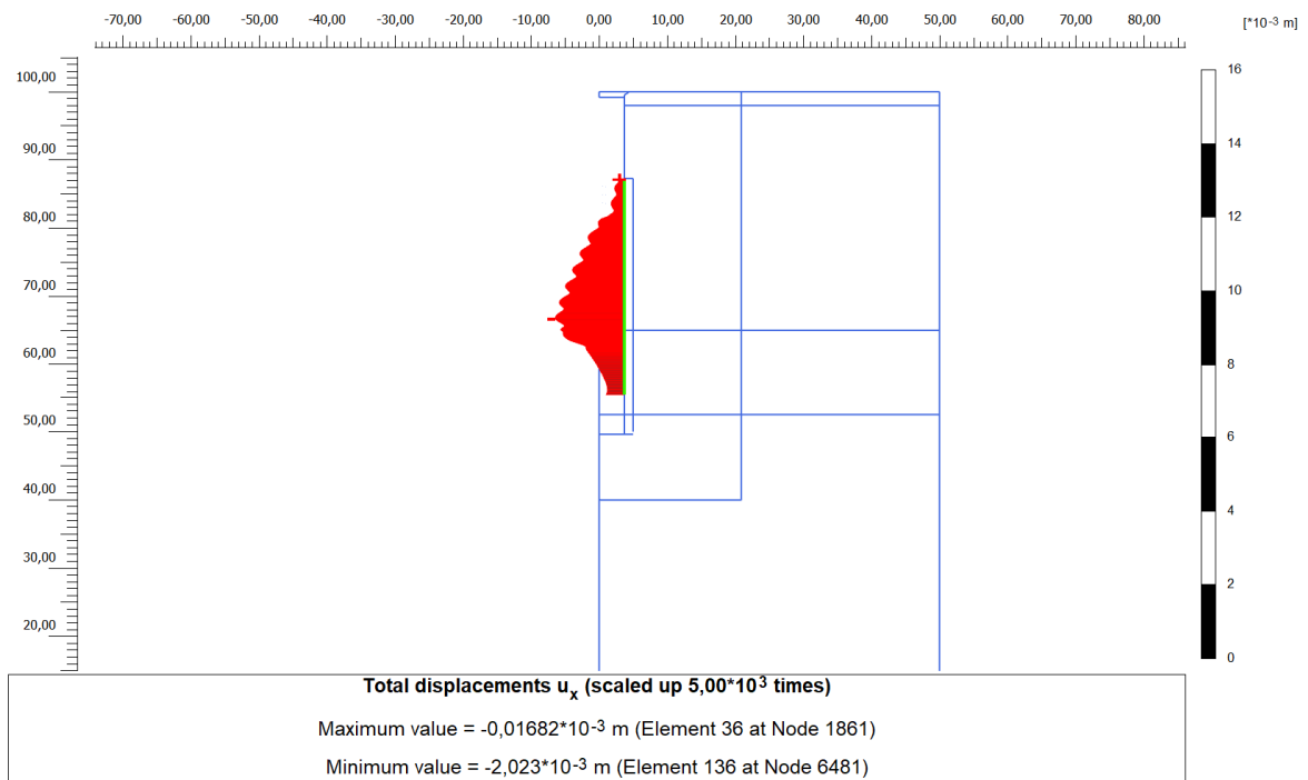
Figura 11. Diagramma degli spostamenti orizzontali della paratia
