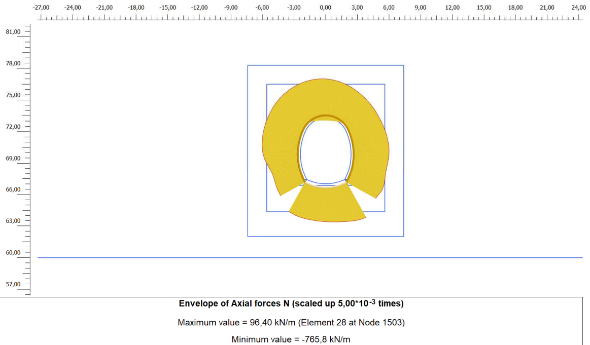
Figura 18. Inviluppo diagramma dello sforzo normale – rivestimento definitivo: Azione sismica (+)
