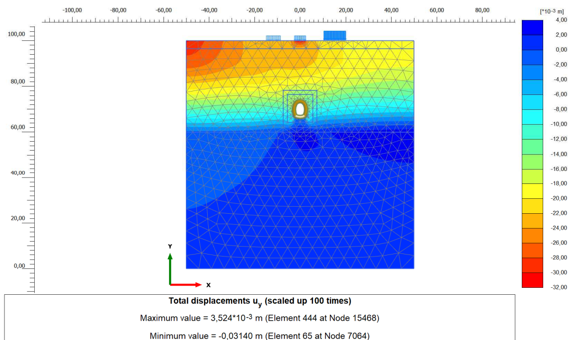
Figura 26. Campo dei cedimenti fase azione sismica (-)
