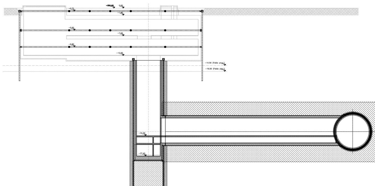
Figura 2. Sezione trasversale del pozzo di ventilazione Pastrengo (PPA)
