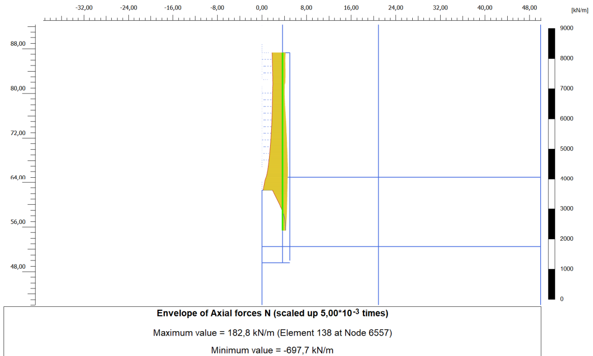
Figura 10. Involuppo dello sforzo normale – SLE
