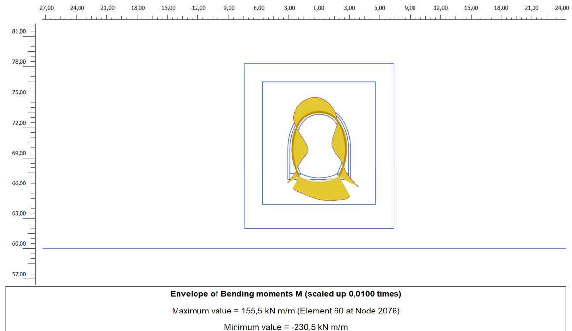
Figura 20. Inviluppo diagramma del momento flettente – rivestimento definitivo: Azione sismica (+)
