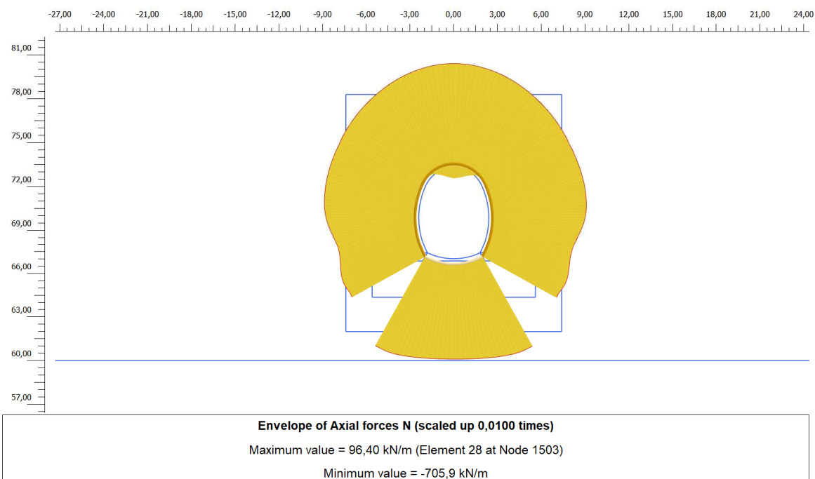
Figura 15. Inviluppo diagramma dello sforzo normale – rivestimento definitivo: Fase di falda a lungo termine
