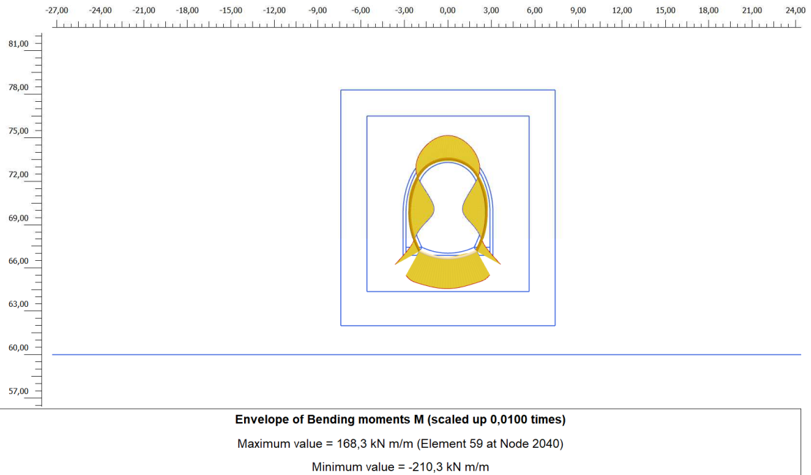
Figura 17. Involuppo diagramma del momento flettente – Rivestimento definitivo: fase di falda a lungo termine
