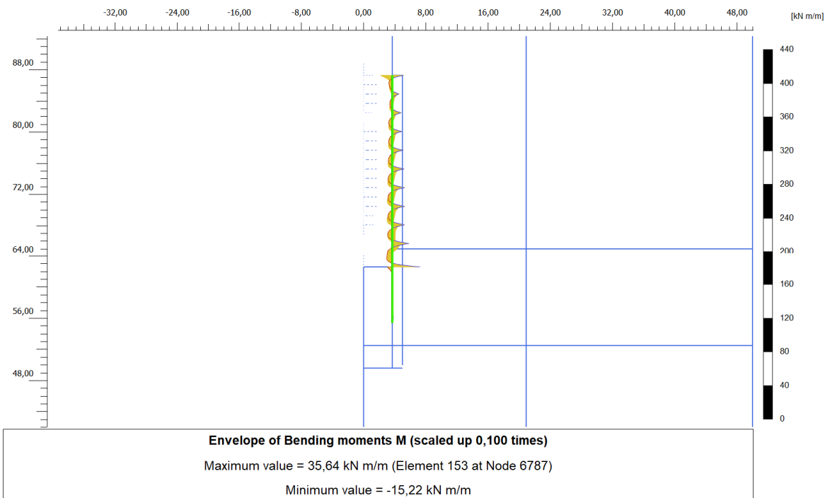
Figura 8. Inviluppo di momento flettente – SLE
