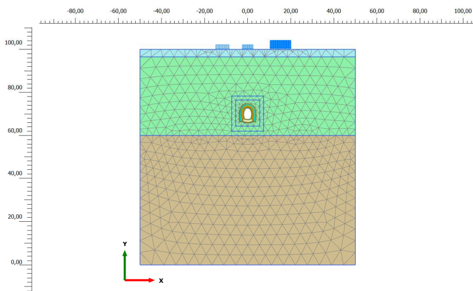
Figura 5. Modello di calcolo e relativa mesh del tronchino di collegamento del pozzo Pastrengo "PPA"
