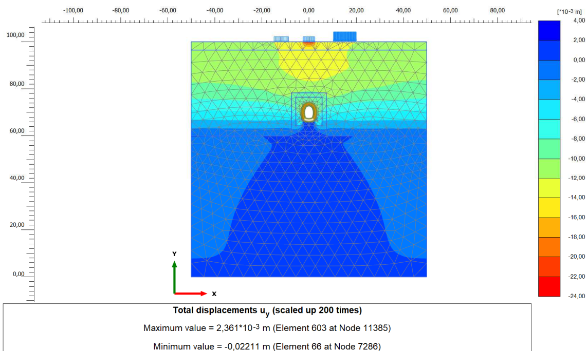
Figura 24. Campo dei cedimenti fase di falda a lungo termine
