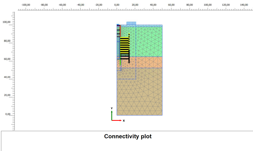
Figura 4. Modello di calcolo e relativa mesh del pozzo Pastrengo "PPA"
