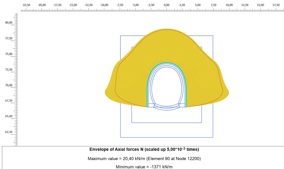
Figura 12. Involuppo diagramma dello sforzo normale - centine
