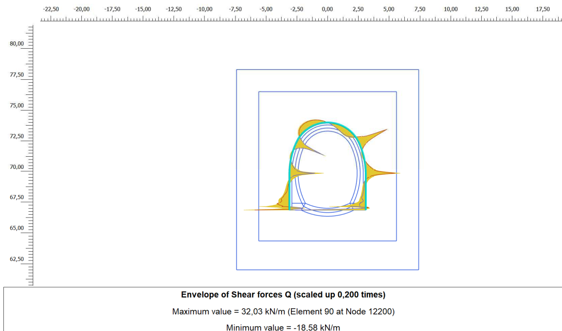
Figura 14. Inviluppo diagramma del taglio – centine
