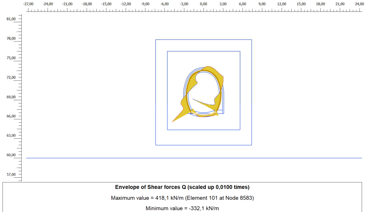
Figura 19. Inviluppo diagramma del taglio – rivestimento definitivo: Azione sismica (+)
