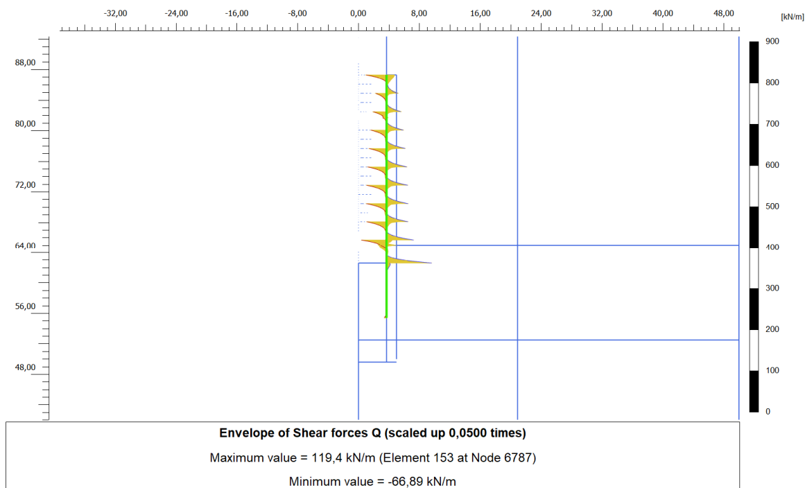
Figura 9. Inviluppo di taglio – SLE
