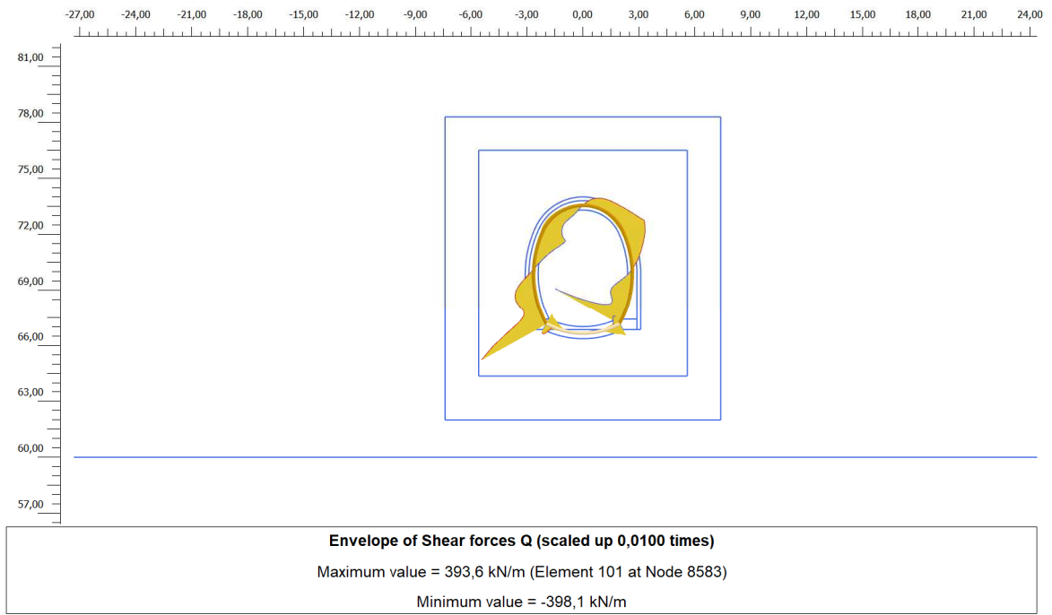
Figura 16. Involuppo diagramma del taglio – rivestimento definitivo: Fase di falda a lungo termine
