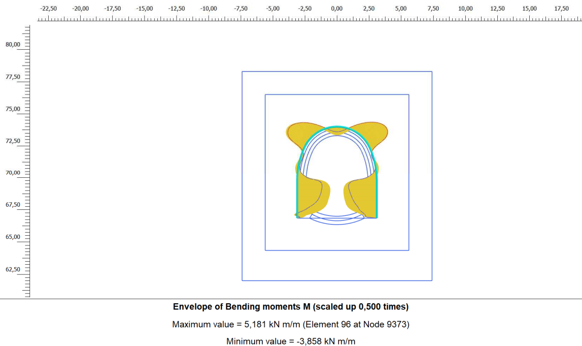
Figura 13. Inviluppo diagramma del momento flettente - centine
