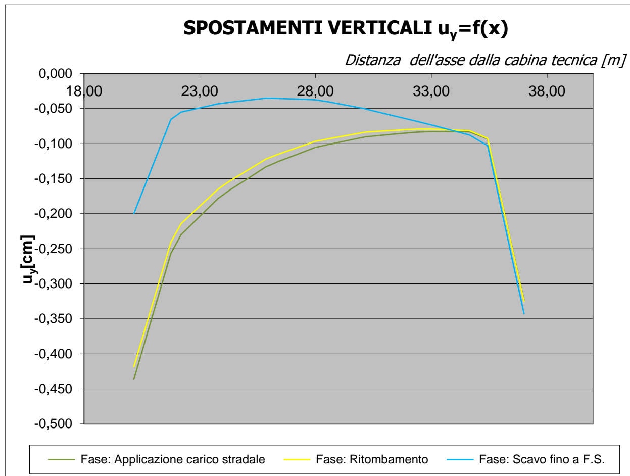
Figura 19. Curva dei cedimenti
