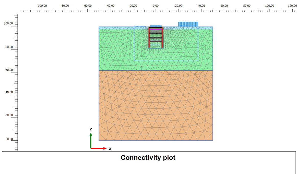
Figura 5. Modello di calcolo e relativa mesh della cabina tecnica di "PCB"
