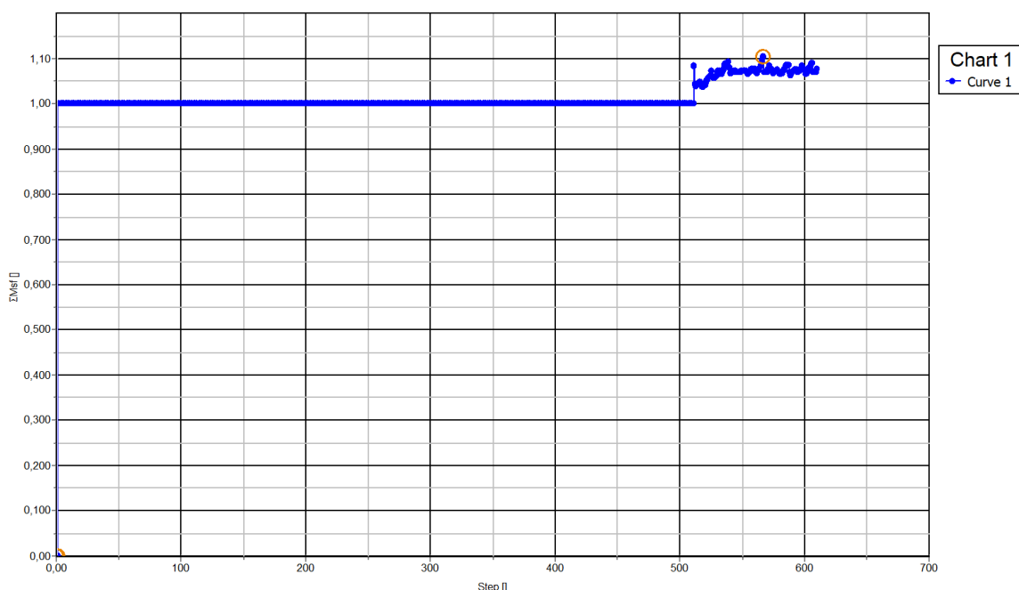
Figura 13. Risultati della Safety Anylisis, fattore di sicurezza
