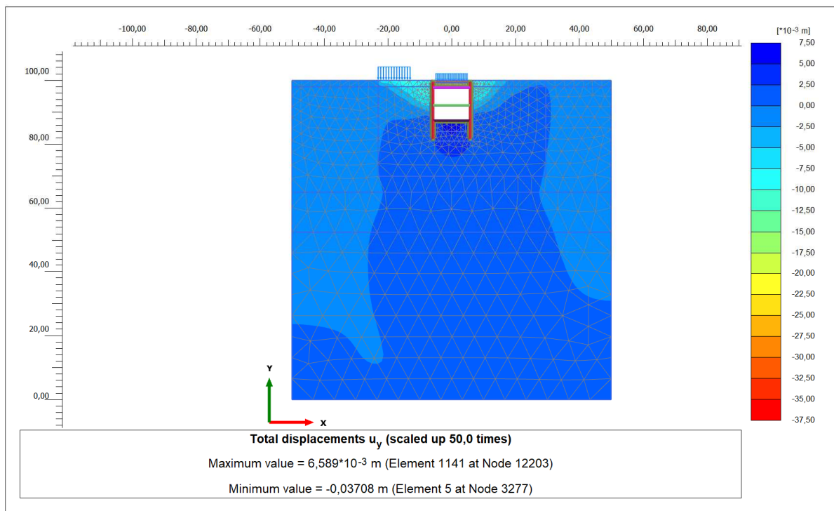
Figura 18. Campo dei cedimenti nel dominio di calcolo discretizzato u_y – Fase (Fase di applicazione del carico stradale)
