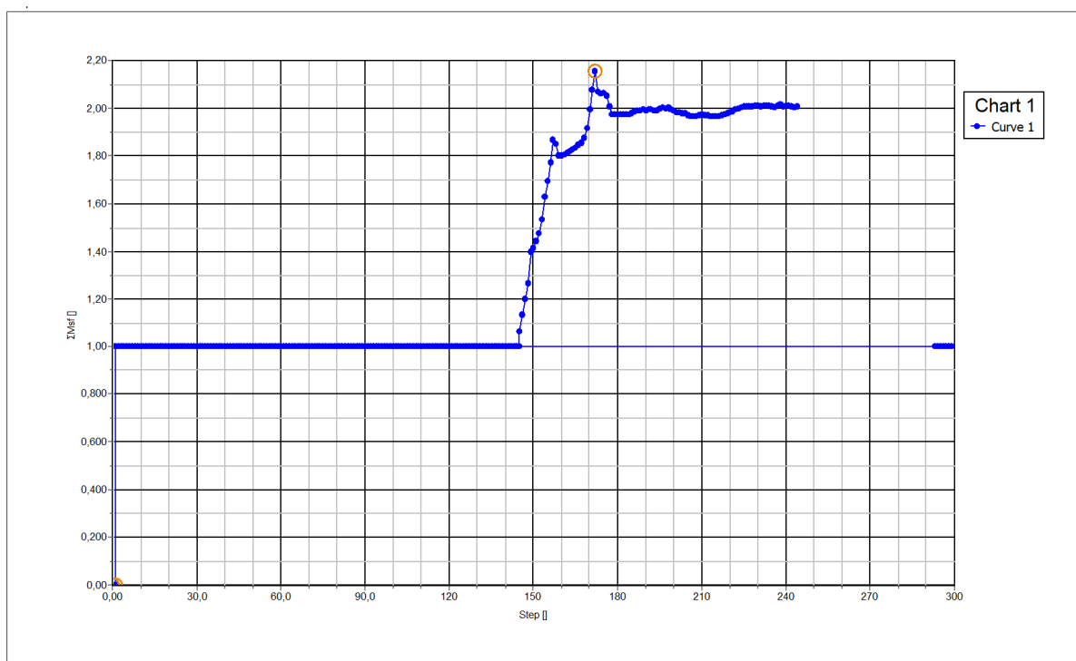
Figura 13. Risultati della Safety Anylisis, fattore di sicurezza
