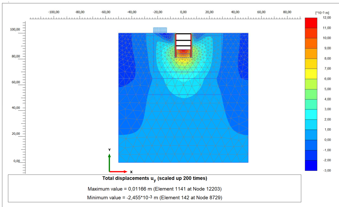
Figura 17. Campo dei cedimenti nel dominio di calcolo discretizzato u_y – Fase (Fase di scavo fino a Fondo scavo)
