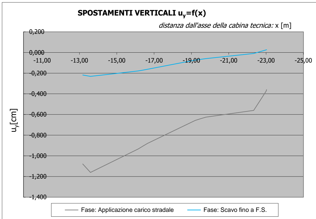
Figura 19. Curva dei cedimenti
