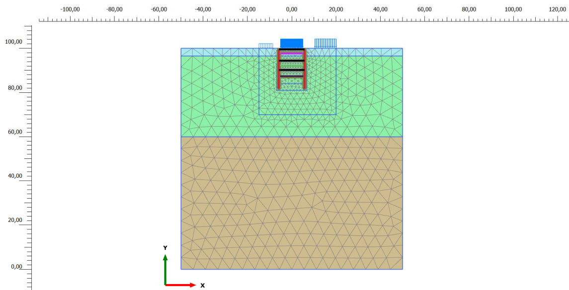
Figura 5. Modello di calcolo e relativa mesh della cabina tecnica di "PPA"
