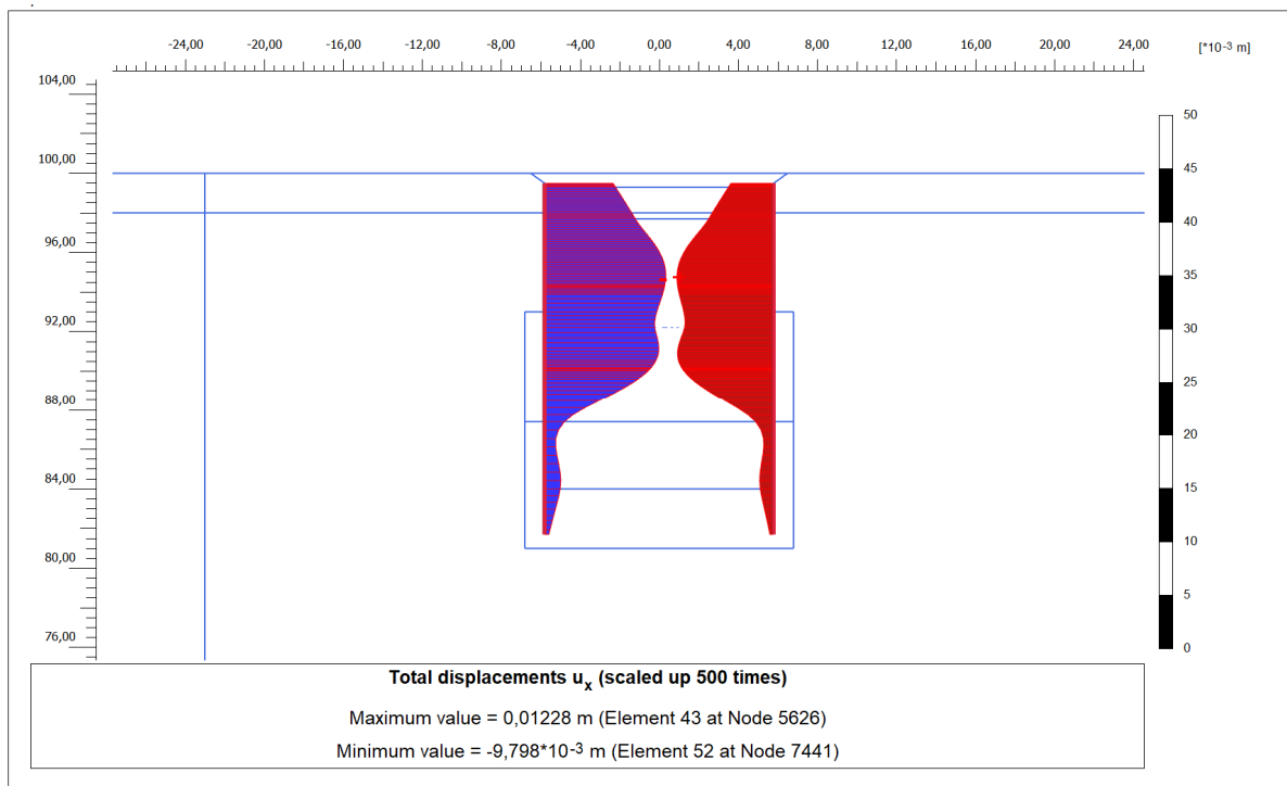
Figura 11. Spostamento massimo orizzontale della paratia
