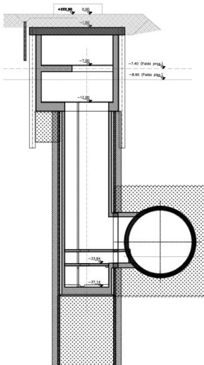
Figura 2. Sezione trasversale del pozzo di ventilazione Mole-Giardini Reali (PMO)
