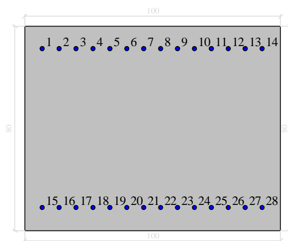
Figura 15. Sezione C.A. tipo di 1.00 m di diaframma
