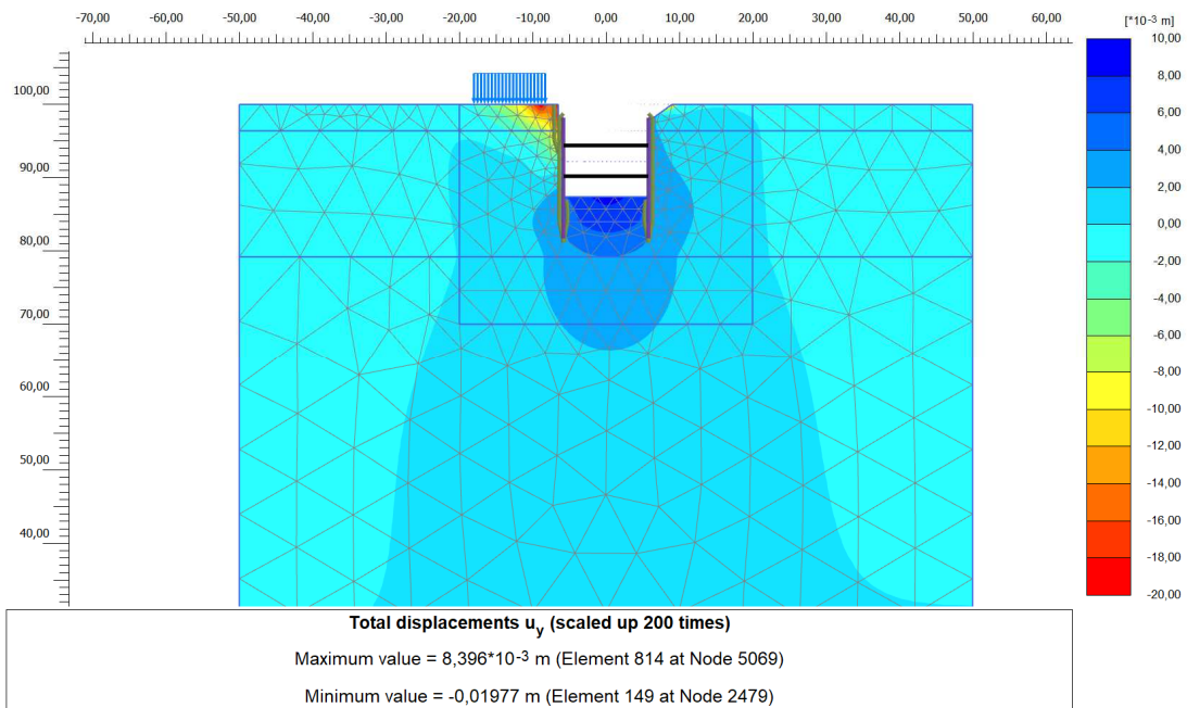
Figura 21. Campo dei cedimenti nel dominio di calcolo discretizzato u_y – Fase 10 (Fase di scavo fino a Fondo scavo)
