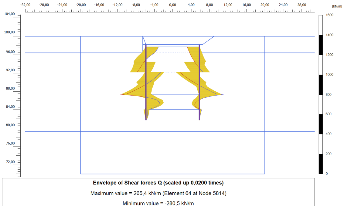
Figura 12. Inviluppo di taglio (considerando una striscia di diaframma pari a 1 m) – SLE
