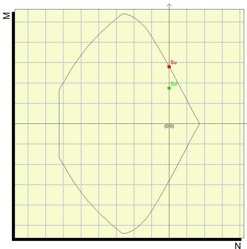
Figura 16. Dominio N-M per la sezione maggiormente sollecitata
