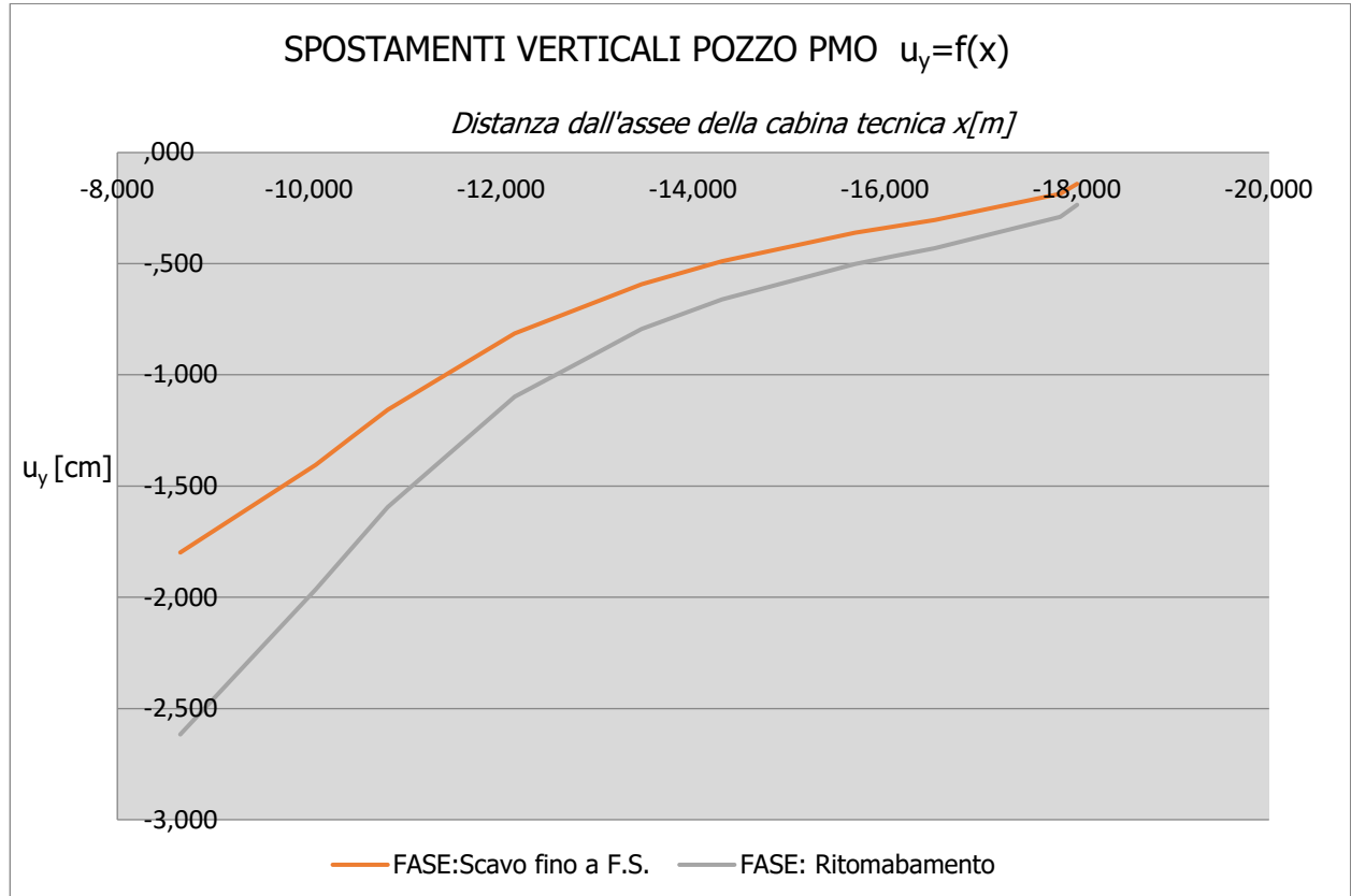
Figura 23. Curva dei cedimenti
