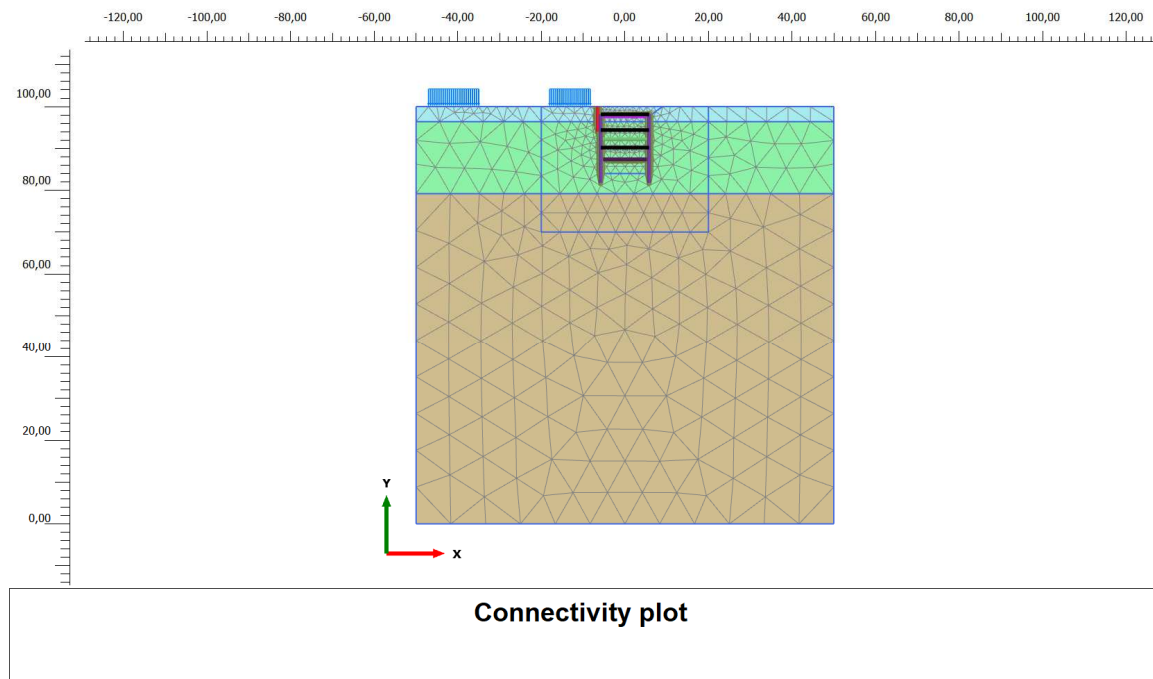
Figura 5. Modello di calcolo e relativa mesh della cabina tecnica di "PMO"
