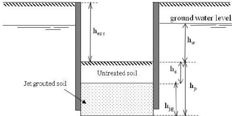
Figura 8. Schema geometrico
