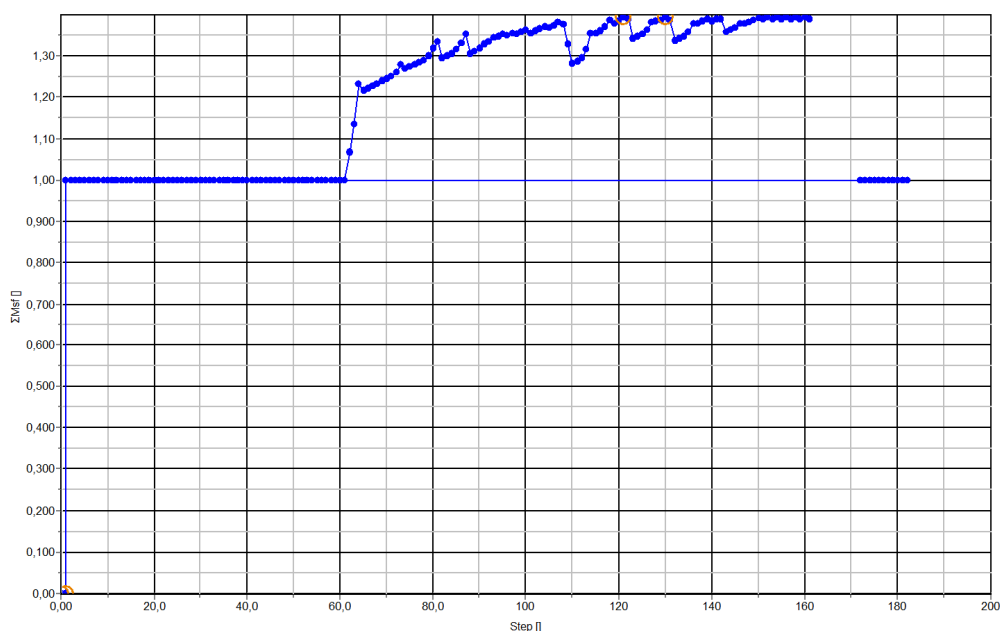
Figura 17. Risultati della Safety Anylisis, fattore di sicurezza
