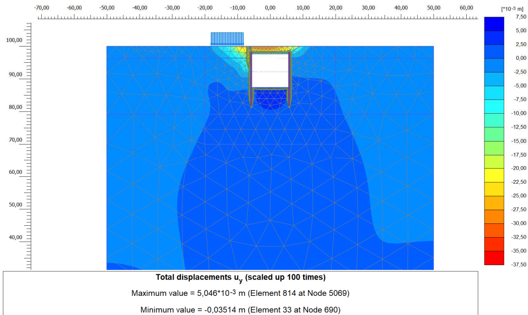
Figura 22. Campo dei cedimenti nel dominio di calcolo discretizzato u_y – Fase 20 (Fase di applicazione del carico stradale)
