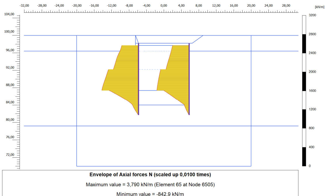
Figura 13. Inviluppo dello sforzo normale (considerando una striscia di diaframma pari a 1 m) – SLE
