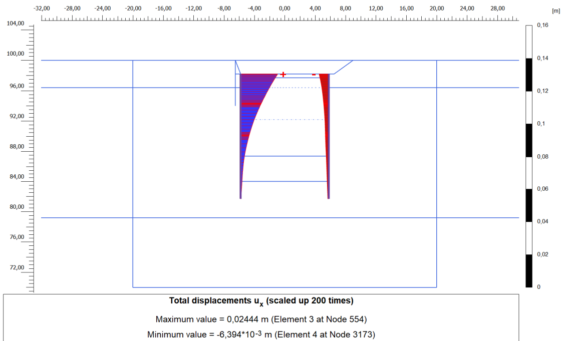
Figura 14. Diagramma degli spostamenti orizzontali dei diaframmi
