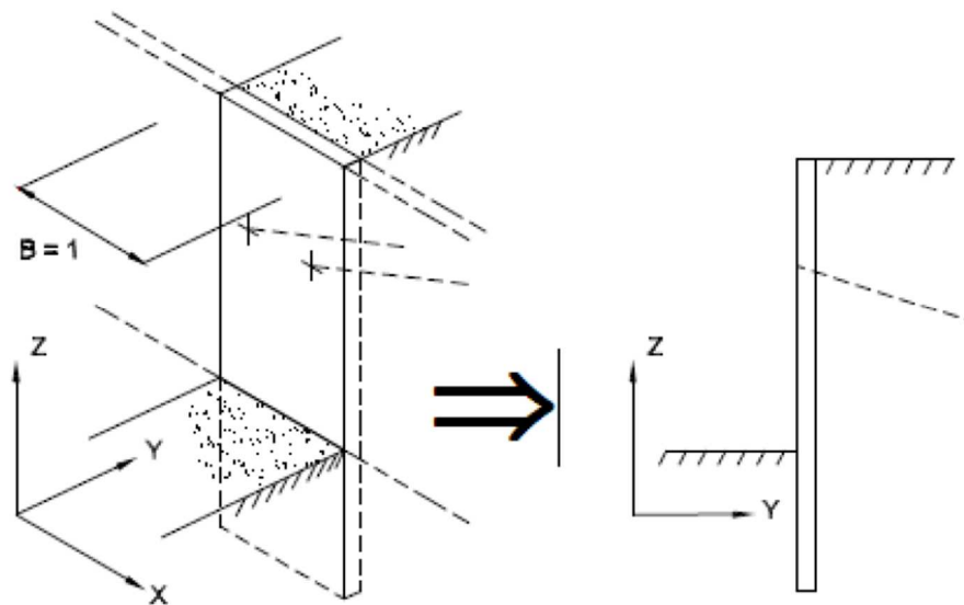
Figura 4. Esempio di modellazione piana della diaframmi
