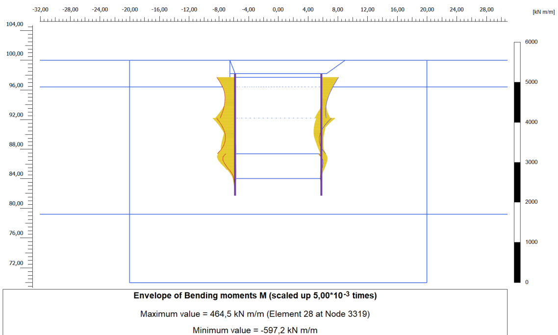
Figura 11. Involuppo di momento flettente (considerando una striscia di diaframma pari a 1 m) – SLE
