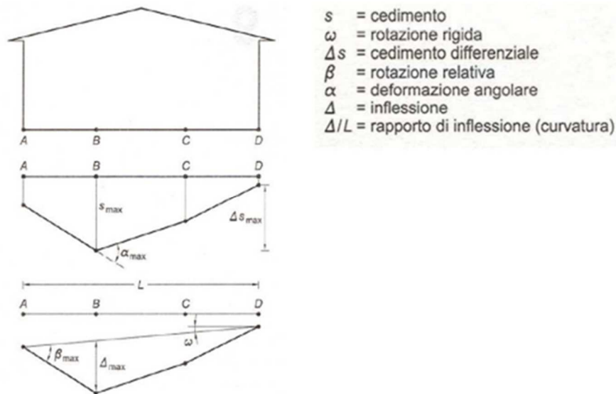
Figura 18. Schema dei parametri di riferimento per la valutazione dei cedimenti
