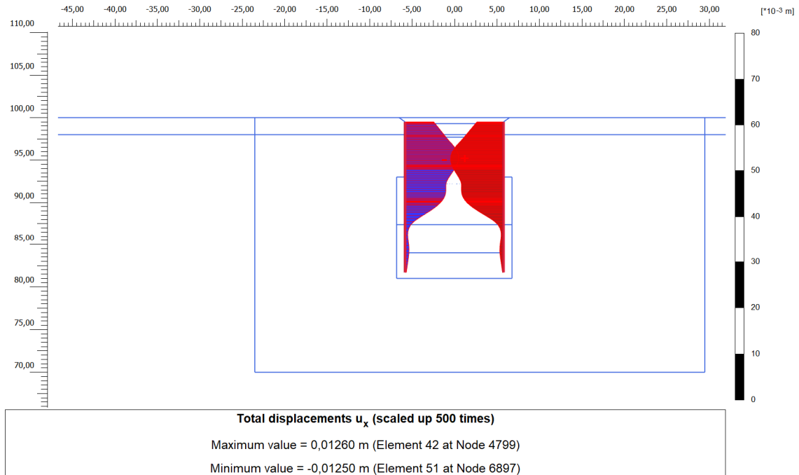
Figura 11. Spostamento massimo orizzontale della paratia
