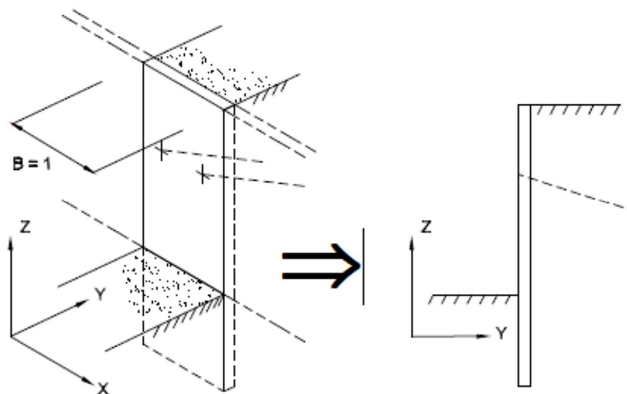
Figura 4. Esempio di modellazione piana della paratia/micropali
