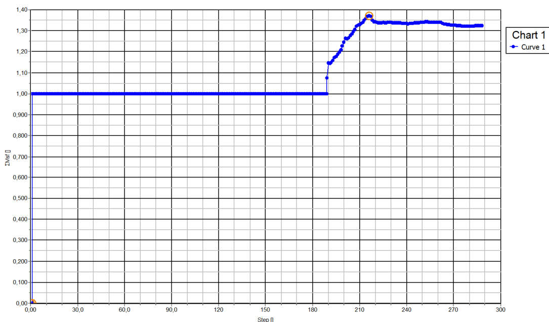
Figura 13. Risultati della Safety Anylisis, fattore di sicurezza
