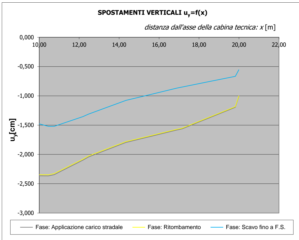
Figura 19. Curva dei cedimenti
