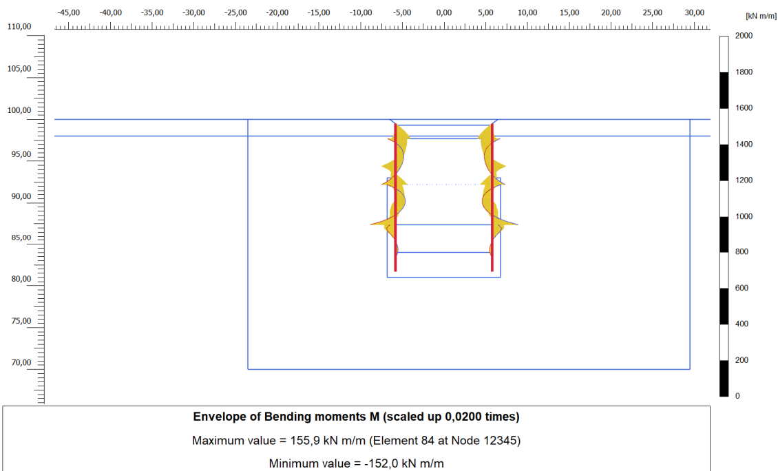
Figura 8. Involuppo di momento flettente (considerando una striscia di paratia pari a 1 m) – SLE
