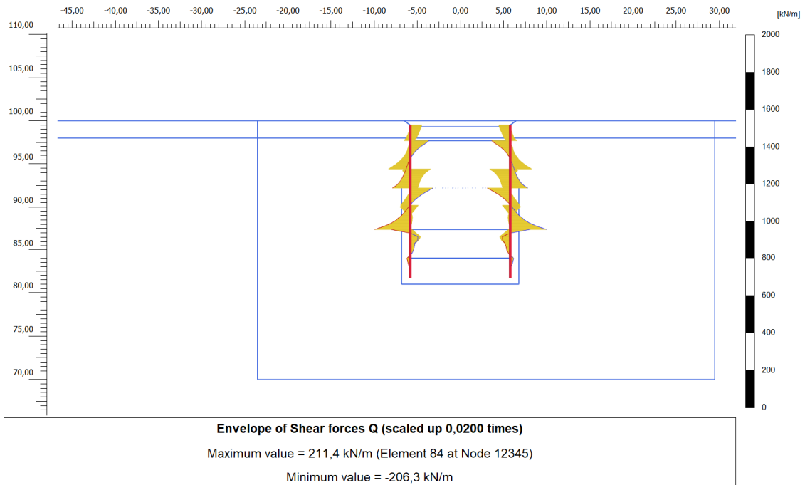
Figura 9. Inviluppo di taglio (considerando una striscia di paratia pari a 1 m) – SLE
