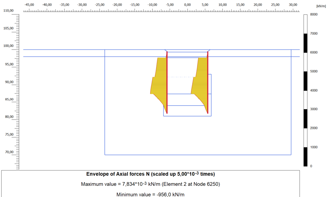
Figura 10. Inviluppo dello sforzo normale (considerando una striscia di paratia pari a 1 m) – SLE
