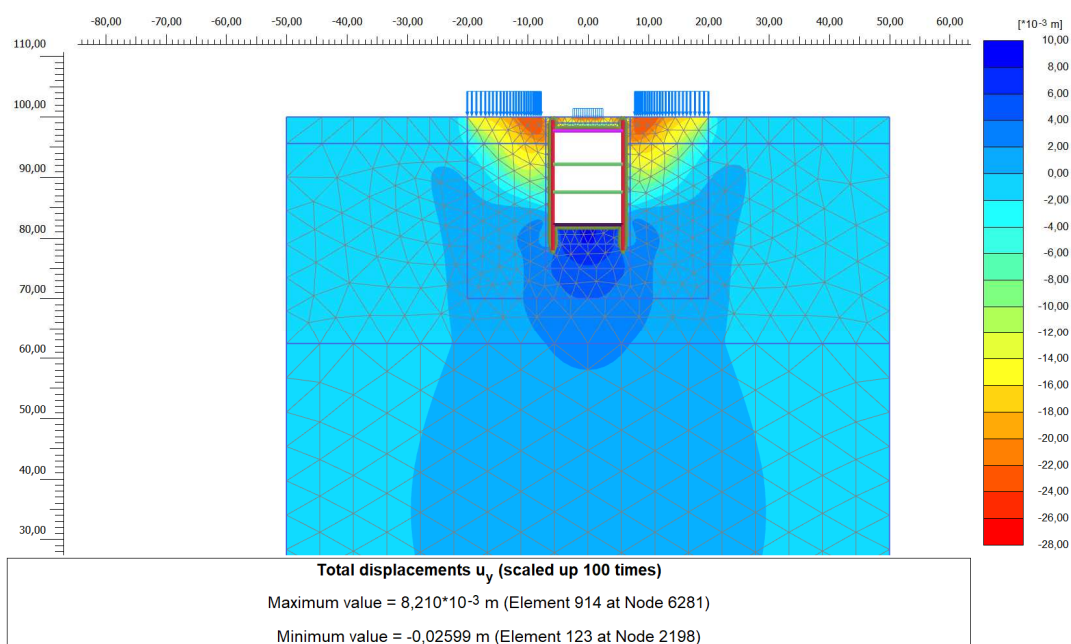
Figura 18. Campo dei cedimenti nel dominio di calcolo discretizzato u_y – Fase 20 (Fase di applicazione del carico stradale)
