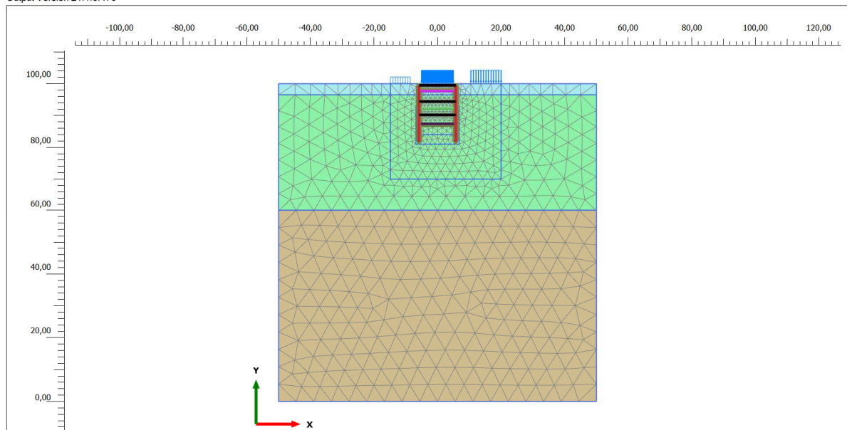
Figura 5. Modello di calcolo e relativa mesh della cabina tecnica di "PCB"
