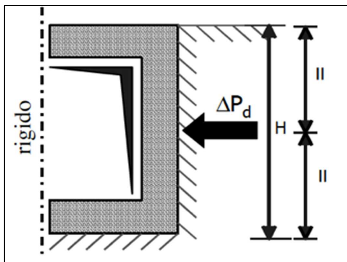
Figura 6. Schematizzazione metodo di Wood
