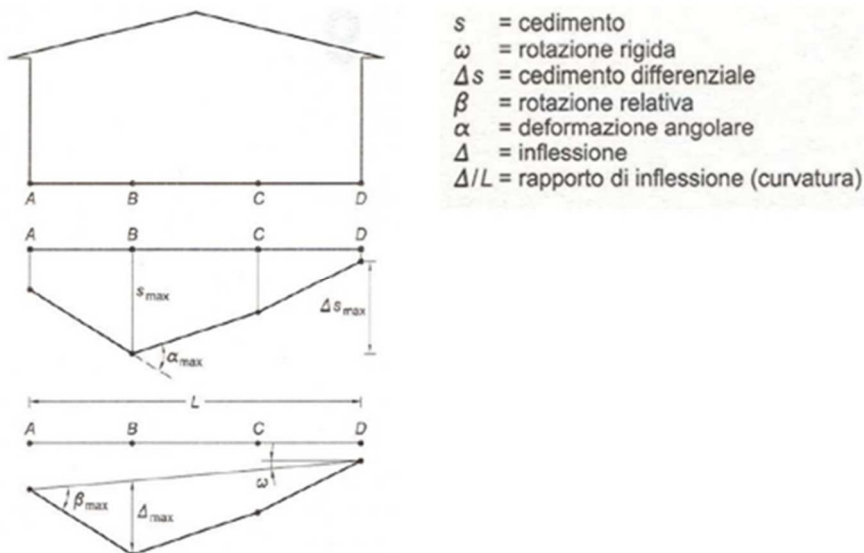
Figura 14. Schema dei parametri di riferimento per la valutazione dei cedimenti
