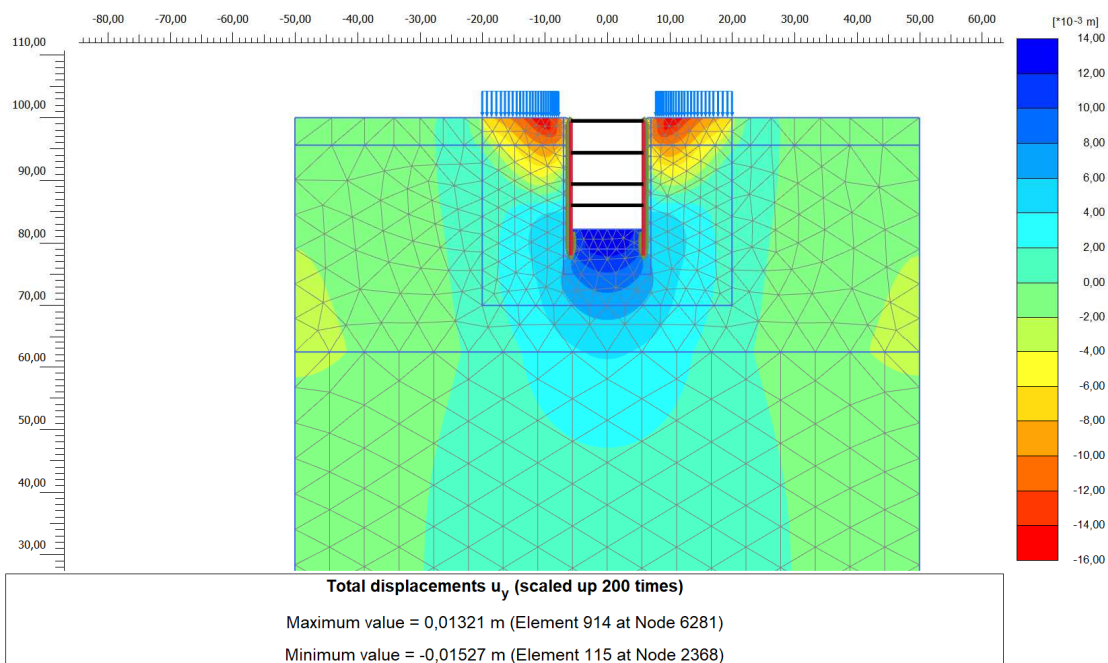
Figura 17. Campo dei cedimenti nel dominio di calcolo discretizzato u_y – Fase 10 (Fase di scavo fino a Fondo scavo)
