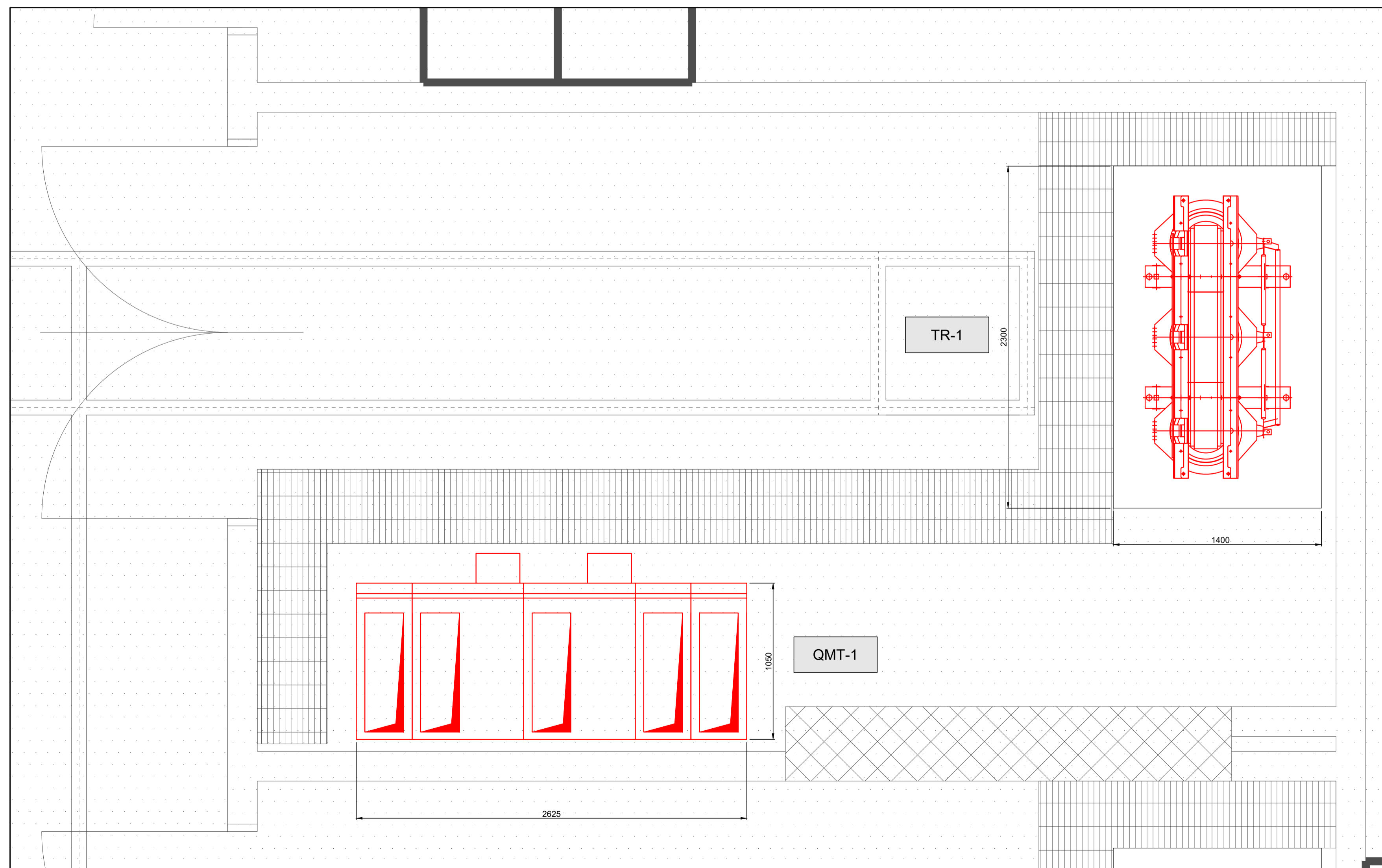
CABINA 1 SCALA 1:20
