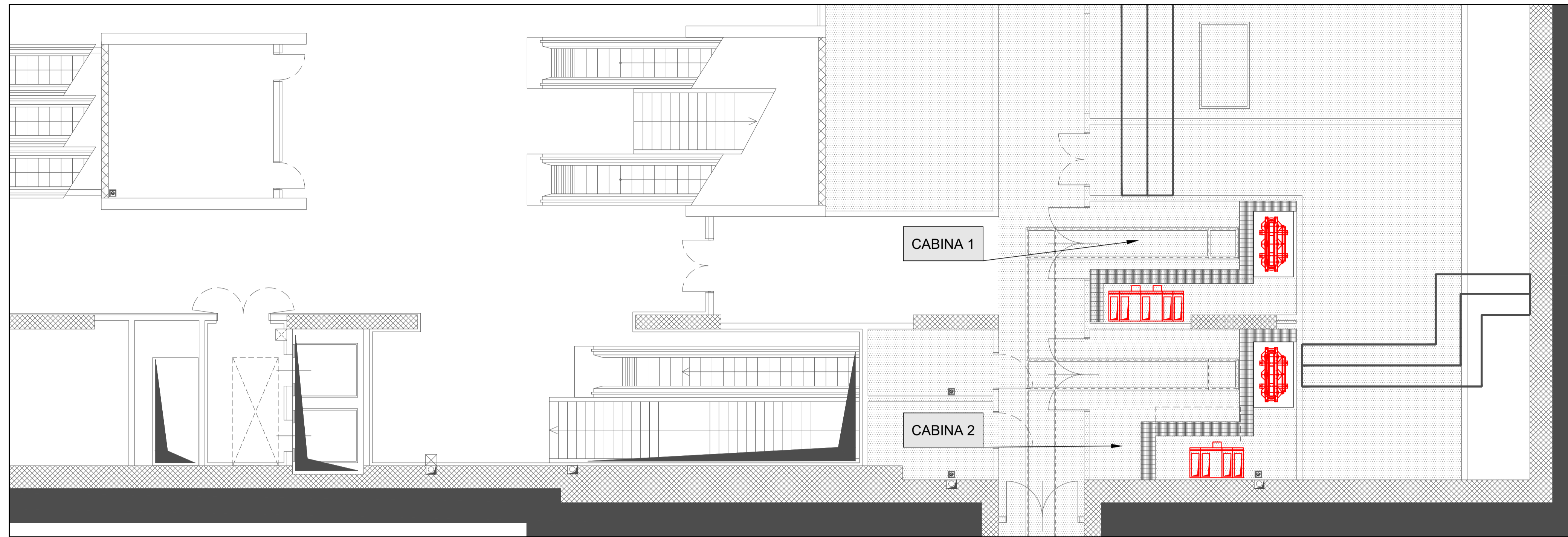
PLANIMETRIA GENERALE SCALA 1:100
