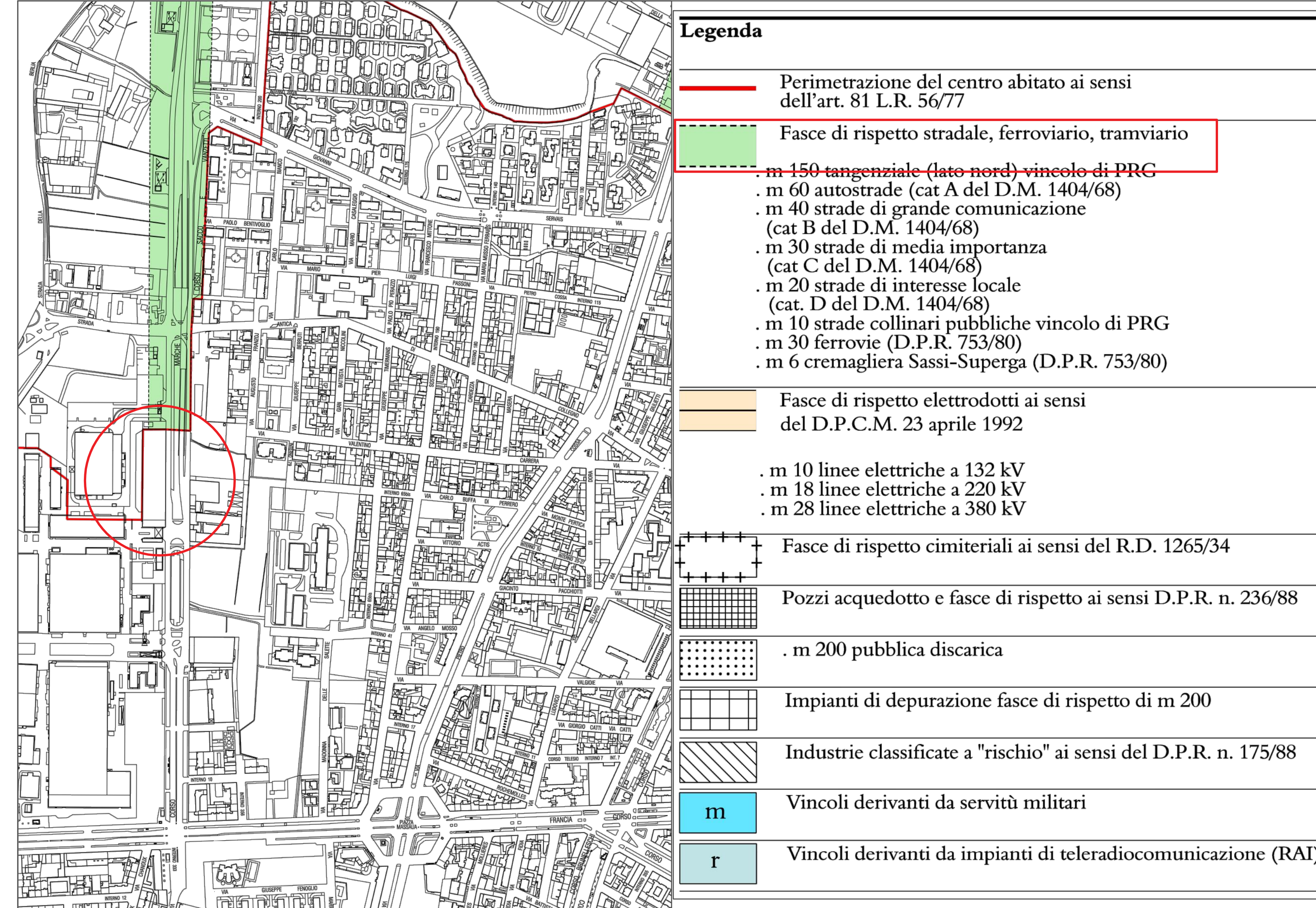
PRGC Torino - Fasce di rispetto Scala 1:5000
