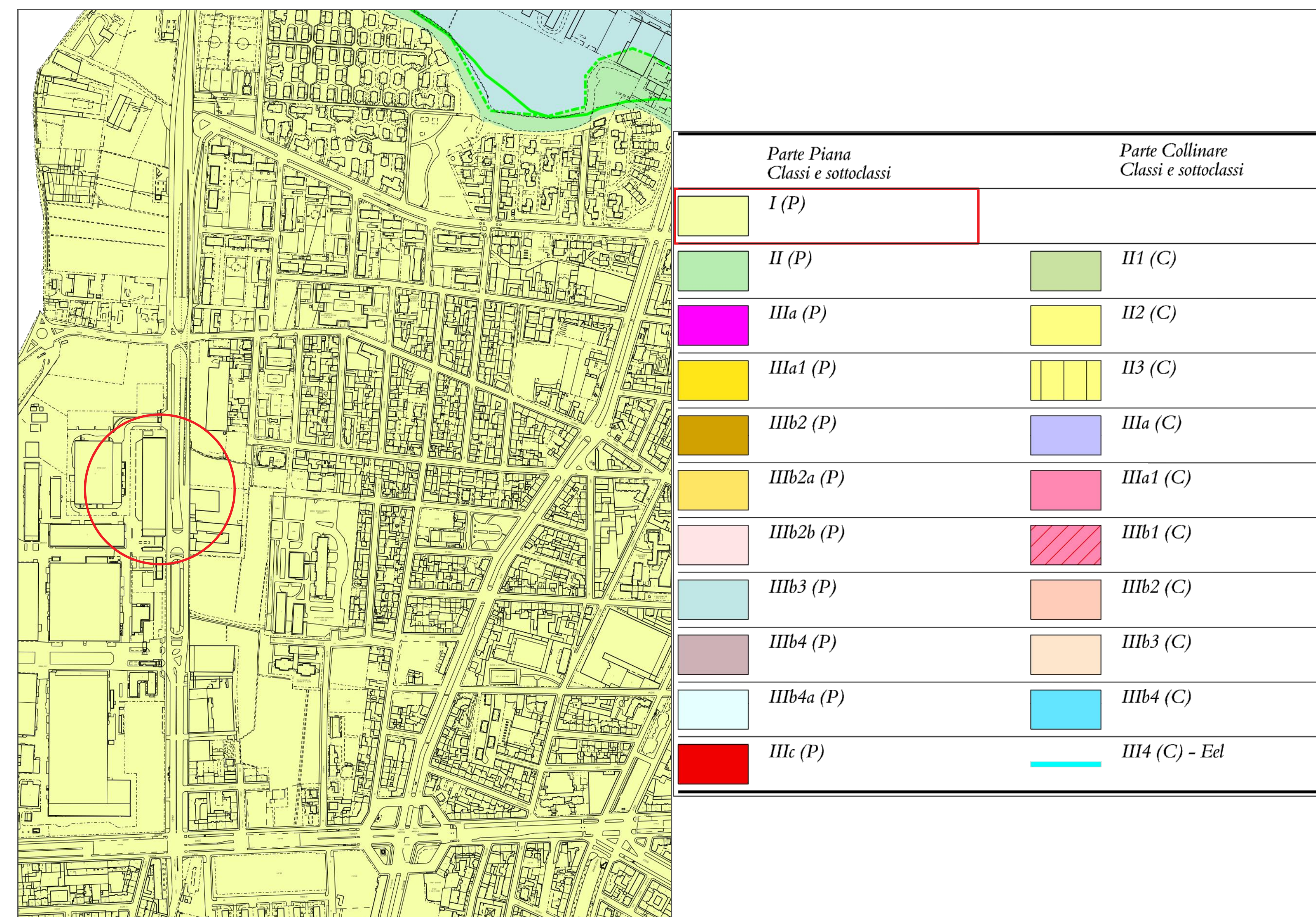
PRGC Torino - Carta di sintesi della pericolosità geomorfologica e dell'idoneità all'utilizzazione urbanistica Scala 1:5000
