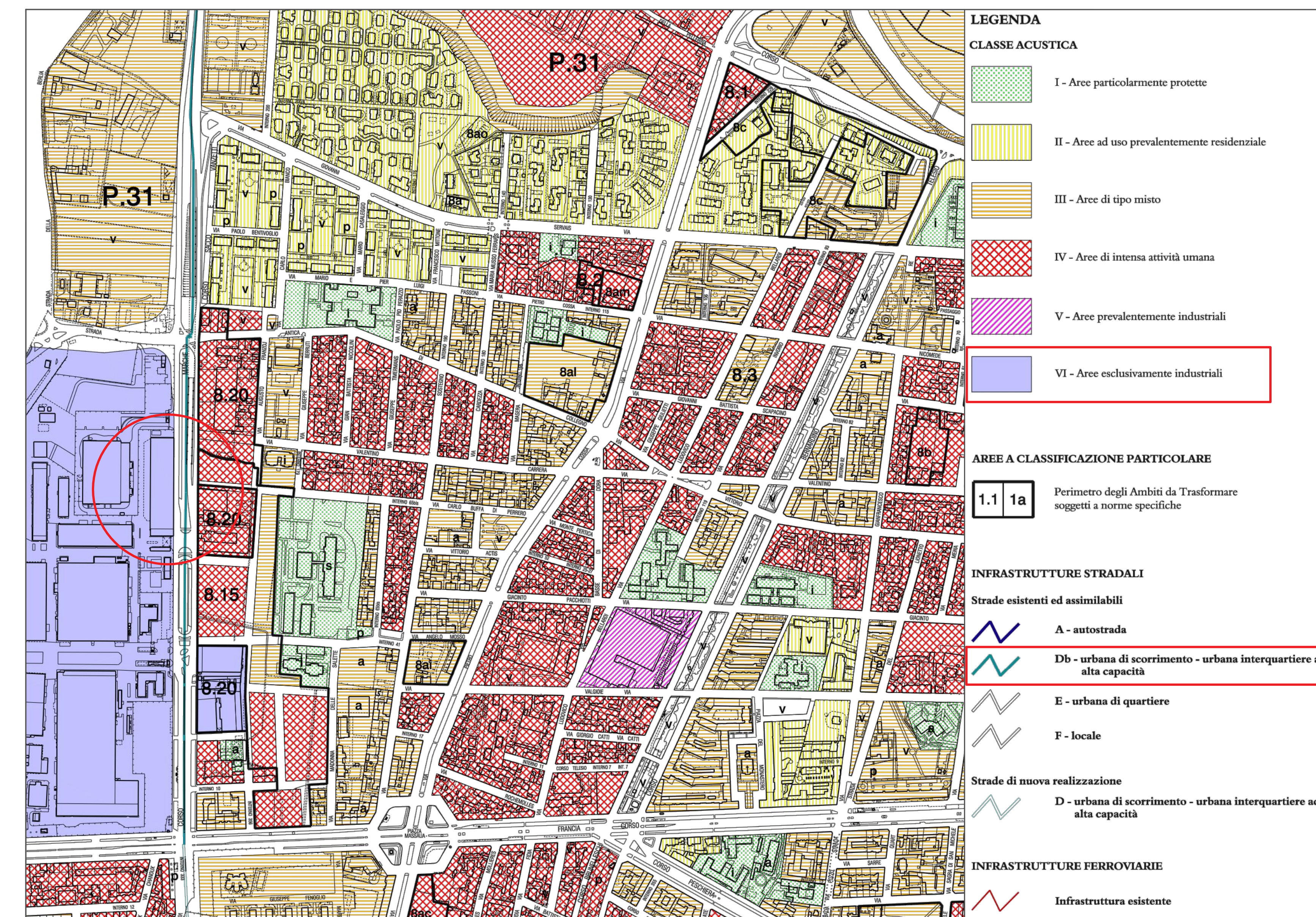
PCA - Fase IV - Inserimento delle fasce "cuscinetto" e delle fasce di pertinenza delle infrastrutture dei trasporti Scala 1:5000
