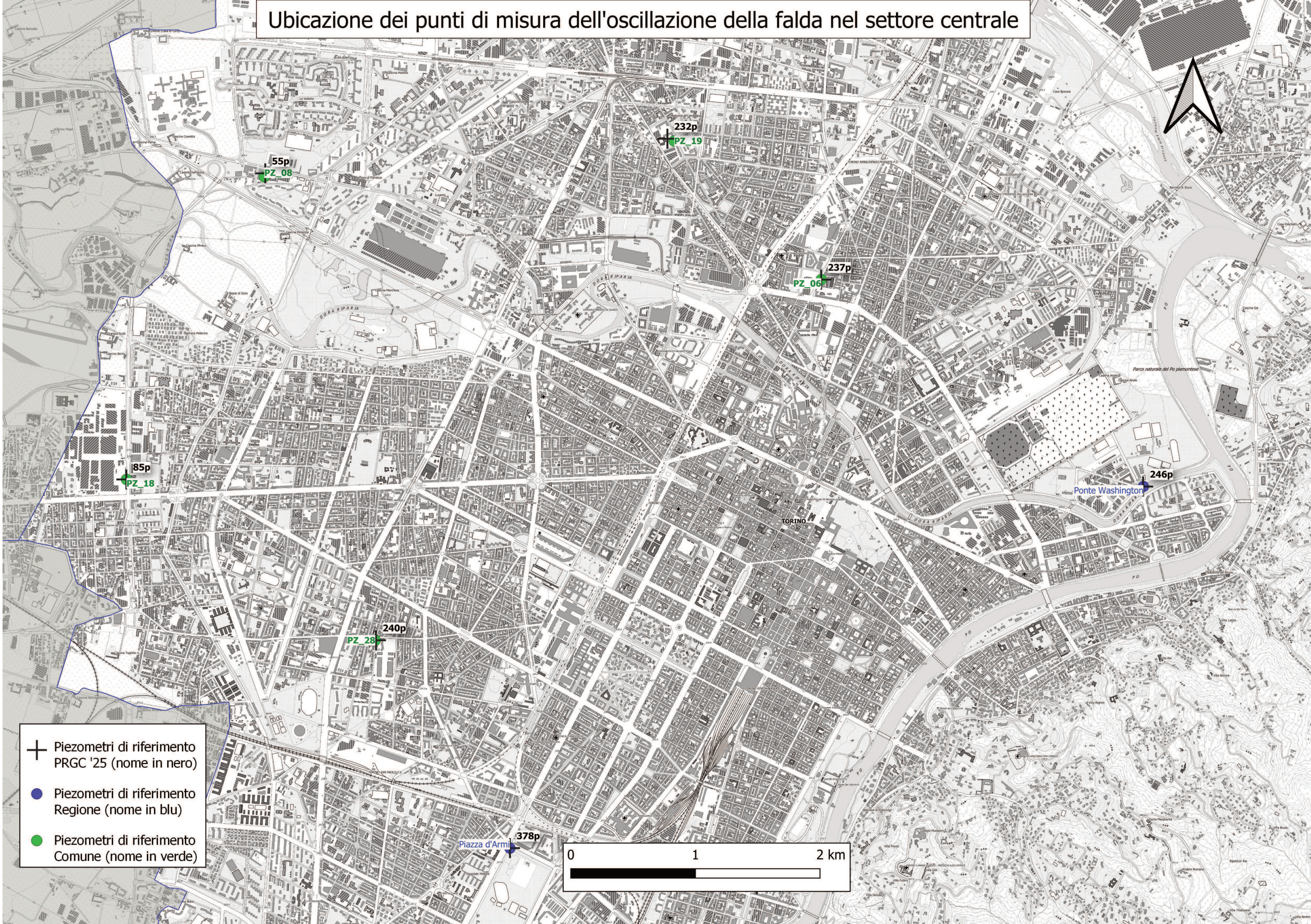
Figura E: confronto tra piezometri Comune e Regione e piezometri PRGC '25 nel settore centro.
