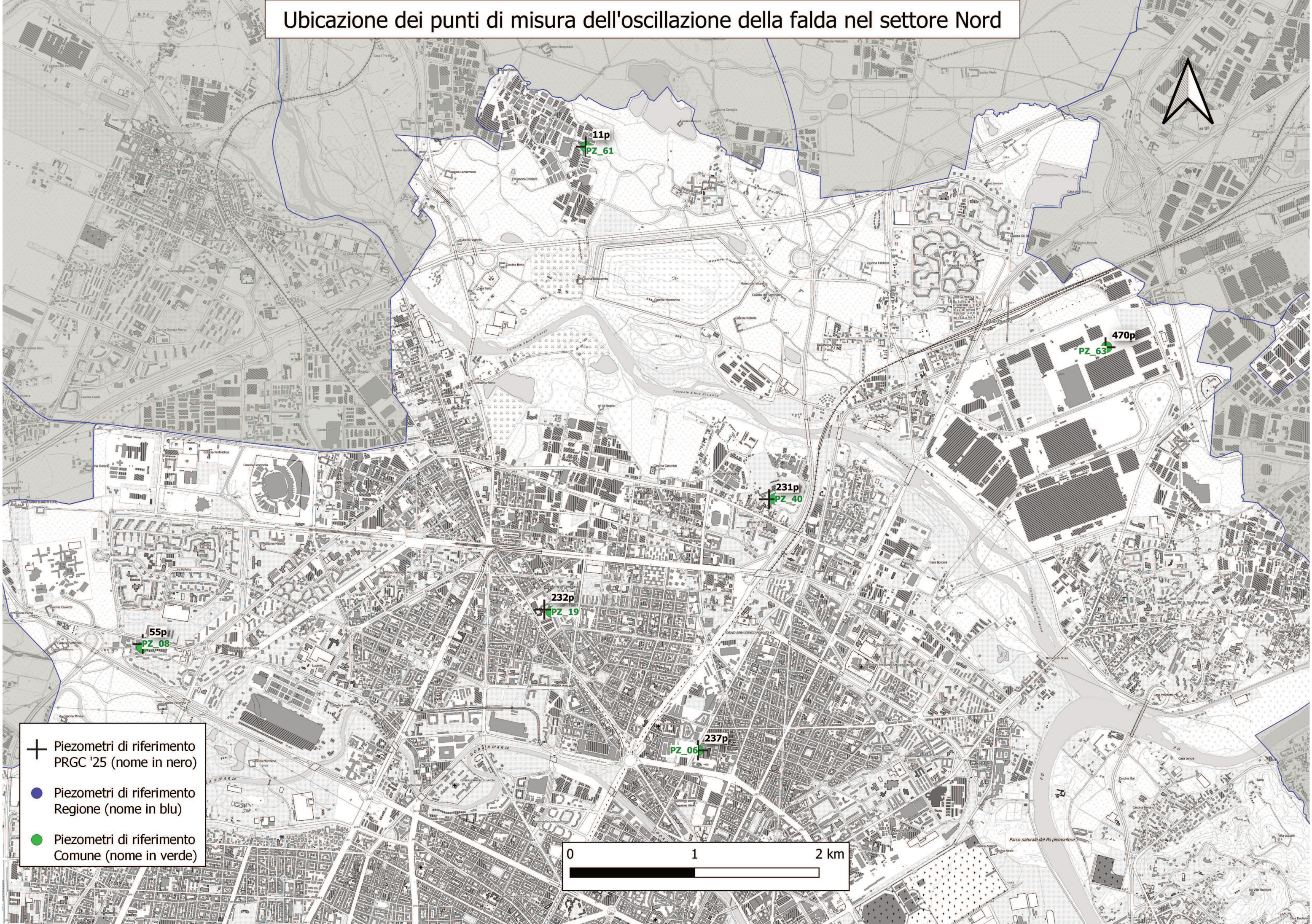
Figura D: confronto tra piezometri Comune e Regione e piezometri PRGC '25 nel settore Nord.
