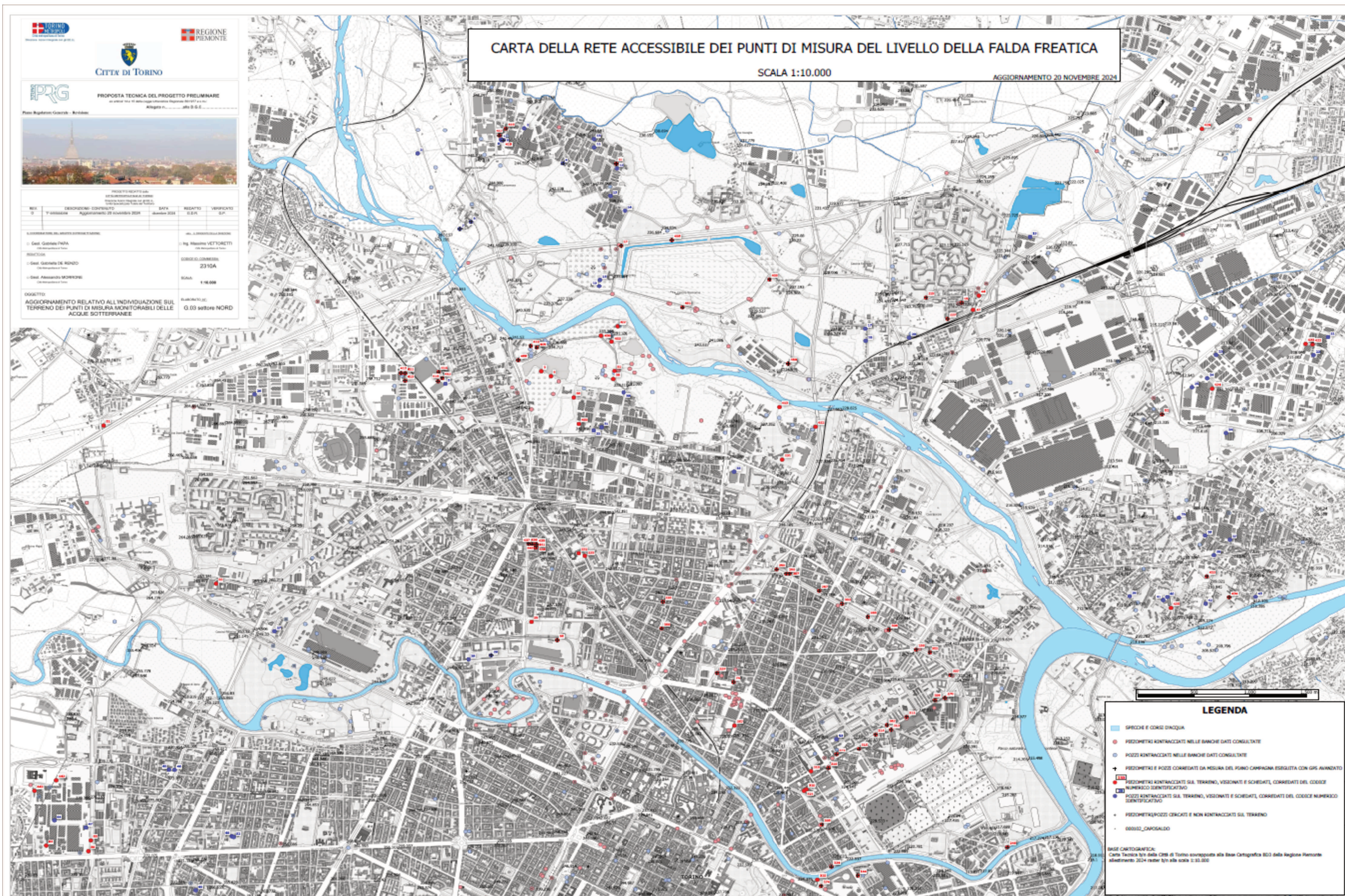
Figura B: Carta "Aggiornamento relativo all'individuazione sul terreno dei punti di misura monitorabili delle acque sotterranee Tavola G03 - Sezione NORD" scala originaria 1:10.000 dicembre 2024
