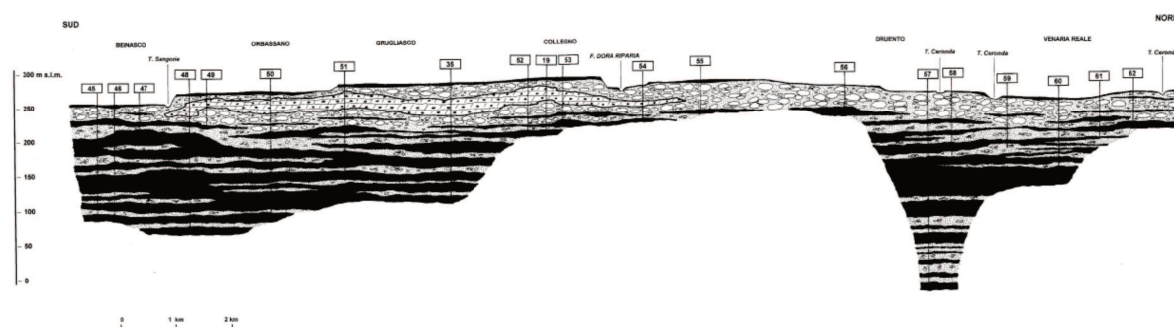
Sezione 6-6' Carta della base dell'acquifero superficiale del settore di pianura della Provincia di Torino
