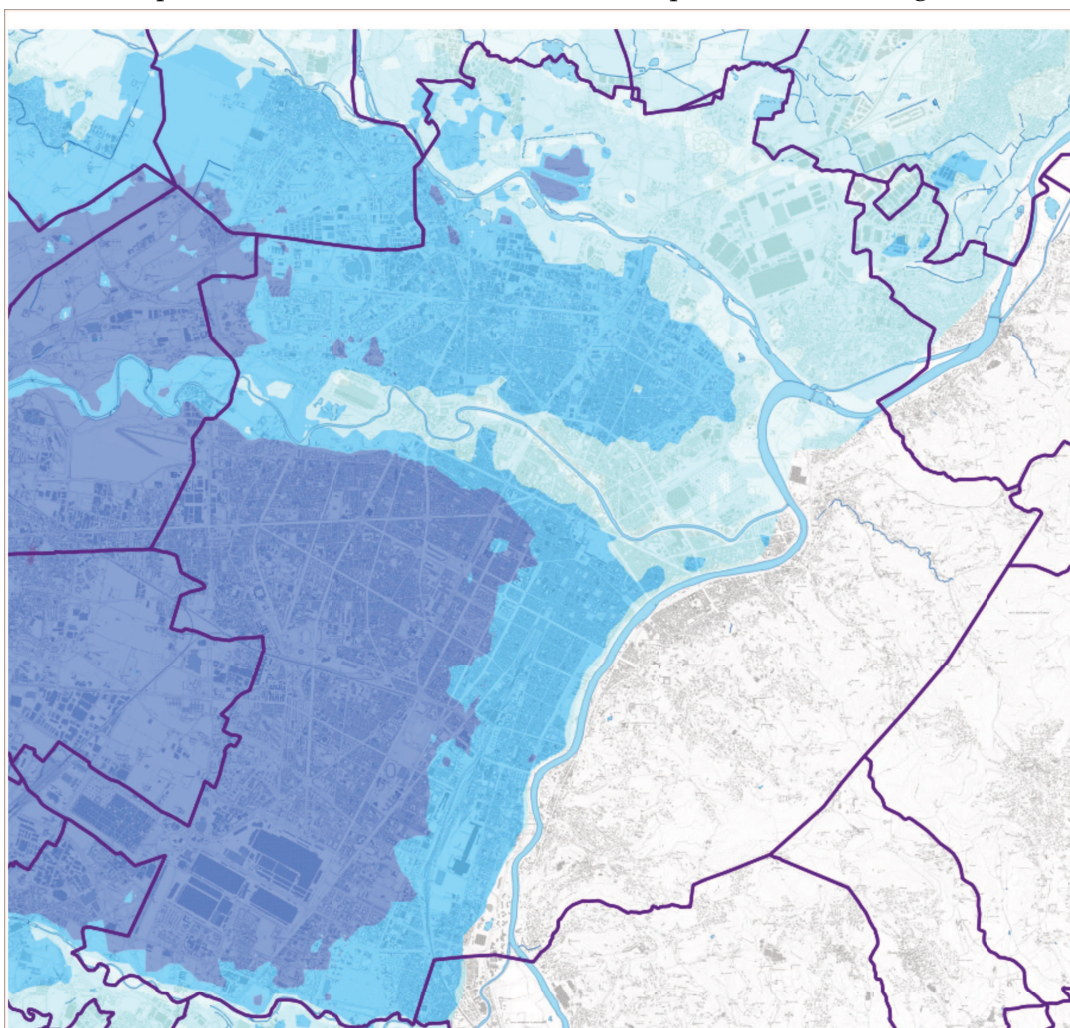
Figura 10: stralcio fuori scala della Carta della soggiacenza di Arpa Piemonte (2002-2005) centrata su Torino. Dal bianco (da 0 a -5 m) al violetto (da -20 a -50) le classi di soggiacenza individuate ogni 5 m
