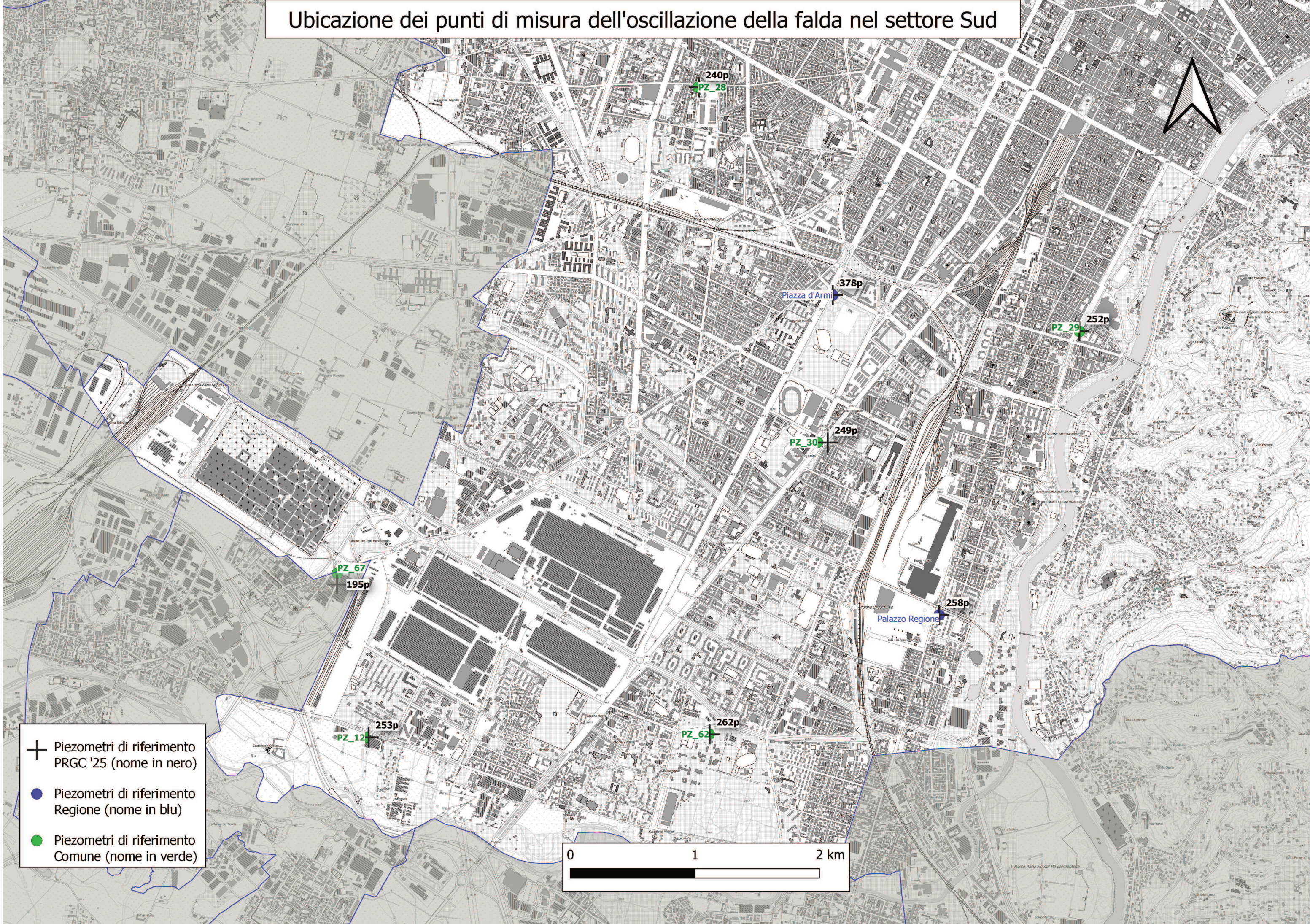
Figura F: confronto tra piezometri Comune e Regione e piezometri PRGC '25 nel settore Sud.
