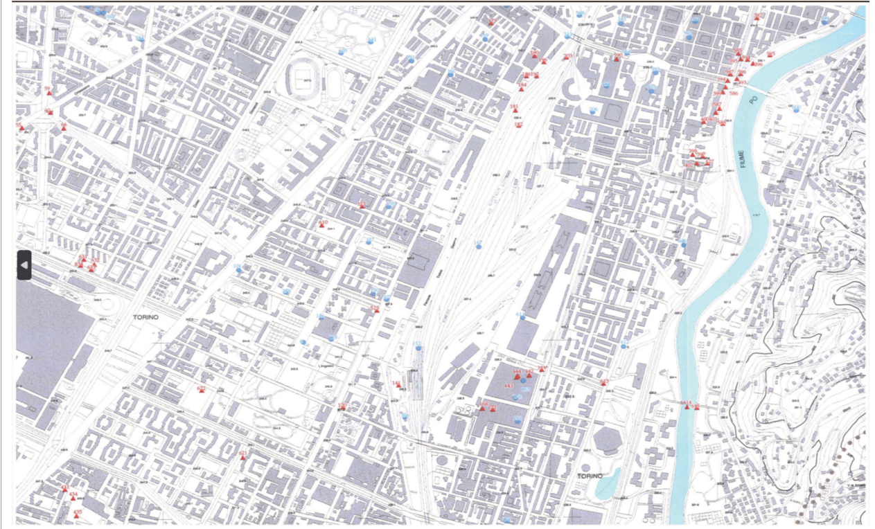
Figura 19: P.R.G.C. Variante 100; stralcio della carta idrogeologica dell'area di pianura Allegato 3-24. I pallini azzurri sono i punti di ubicazione dei pozzi muniti di stratigrafia e i triangolini rossi sono i punti di ubicazione dei sondaggi, entrambi con il relativo numero di riferimento
