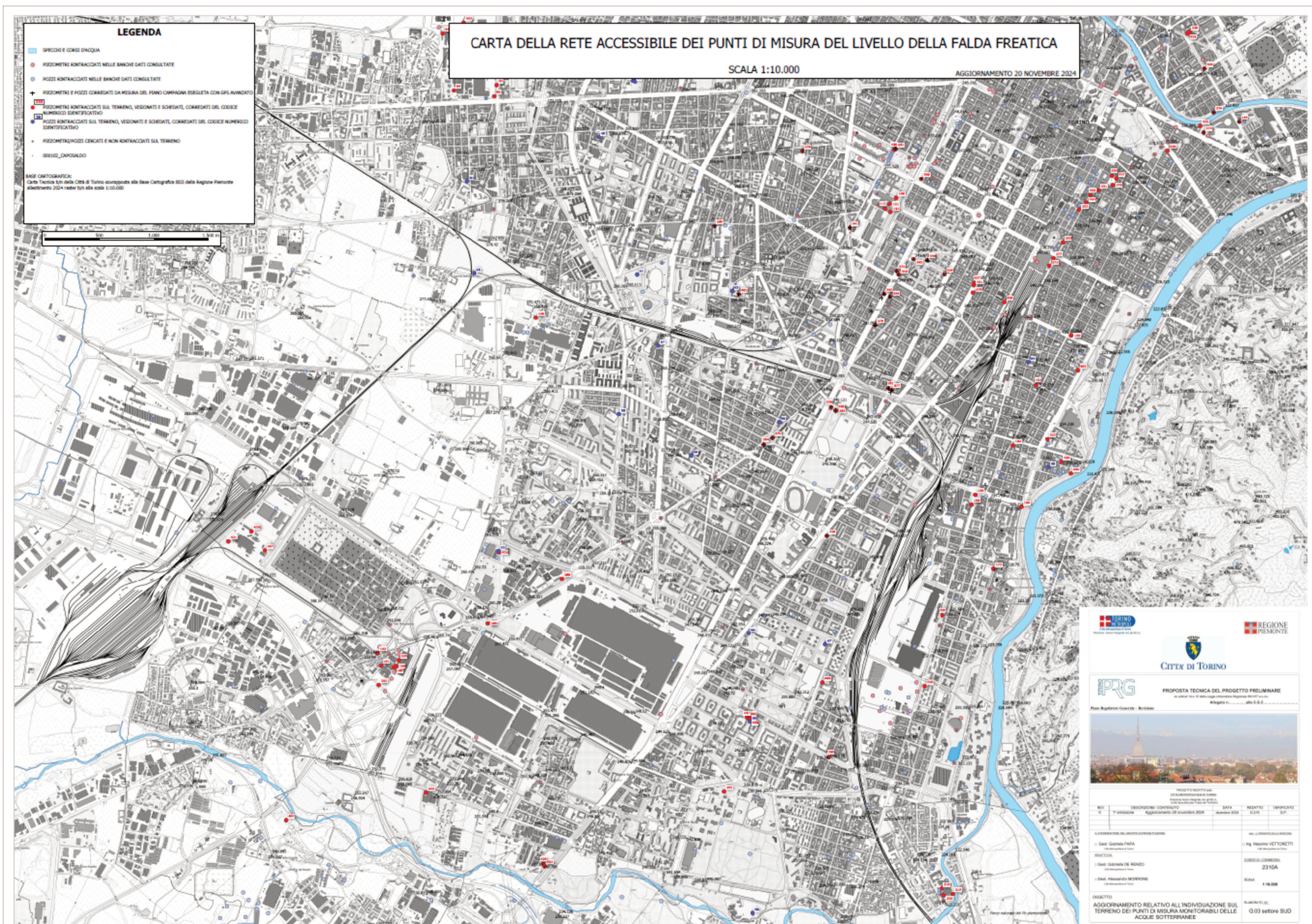
Figura C: Carta “Aggiornamento relativo all’individuazione sul terreno dei punti di misura monitorabili delle acque sotterranee – Tavola G03 – Sezione SUD ” scala originaria 1 : 10.000 dicembre 2024
